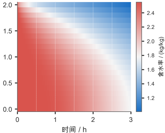
(b) 水分浓度场 C(r, t)
