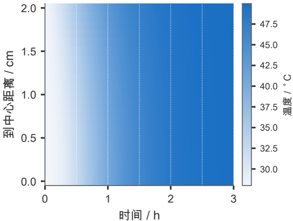
(a) 温度场 T(r, t)
