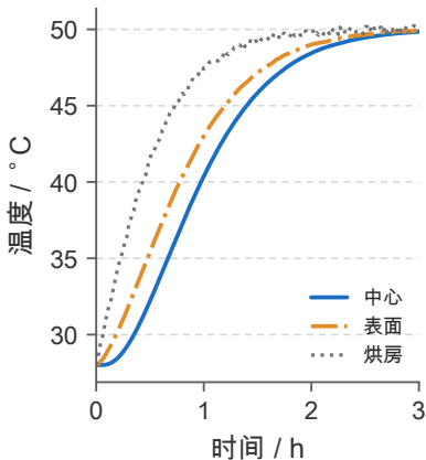
(a) 温度快速趋于均匀
