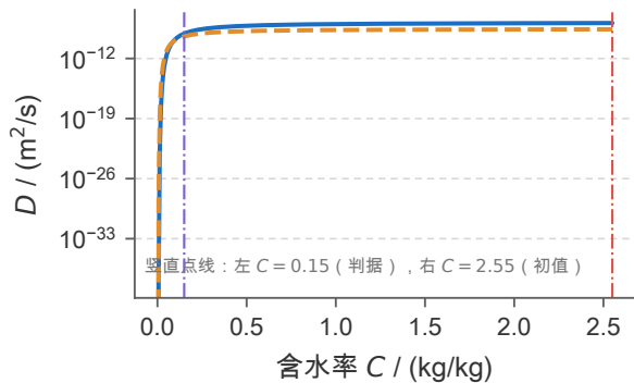
(d) 水分扩散系数
