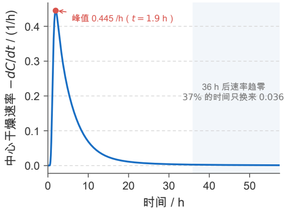
(a) 干燥速率的时间历程
