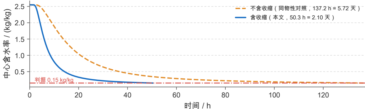
(b) 忽视收缩把烘干时长高估约 2.73 倍
