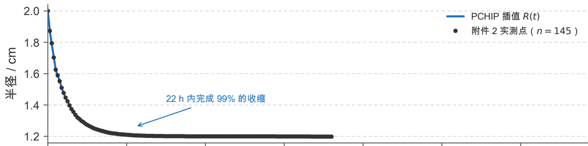
(b) 忽视收缩把烘干时长高估约 2.73 倍
