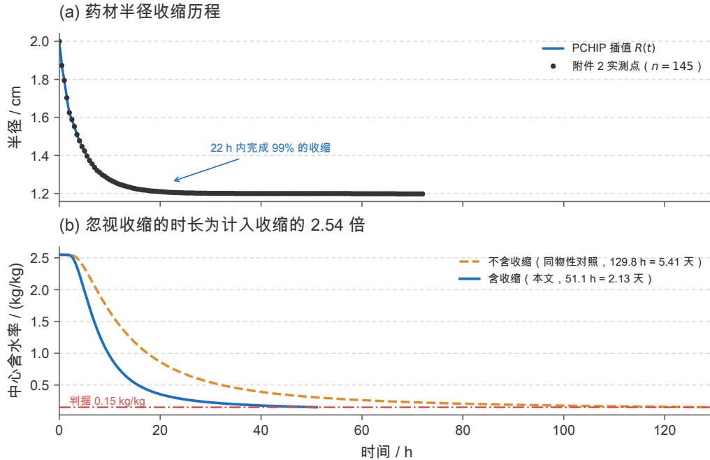
图 8 问题四：收缩历程与烘干时长的对照（附录 4 物性， N = 200 、 \Delta t = 5 s）。(a) 附件 2 的实测半径（ n = 145 ，间隔 1800 s，实测点以散点示出）与保单调三次 Hermite 插值曲线；插值后 \dot{R} \leq 0 恒成立、无过冲。(b) 中心水分浓度随时间的变化：含收缩时 51.08 h 达标，固定半径的对照工况需 129.79 h，收缩使烘干时长缩短约 61%。两图均为确定性数值结果，不含统计误差。
