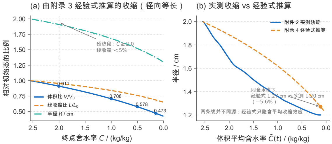
图9 (a)由附录3经验式推算的几何收缩：体积比 V/V_0 、线收缩比 L/L_0 与对应半径随终点含水率的变化； C \geq 2.0 时线收缩不足5%（径向等长口径）。(b)由 \rho(C) 反推的 R(C) 与附件2实测 R-C 轨迹的对照（横轴为体积加权平均含水率 \bar{C} ）：同一含水率下经验式比实测偏大约5.6%，外推到绝干则只差1.1%；路径上前者与含水率同步、后者高度前置。
