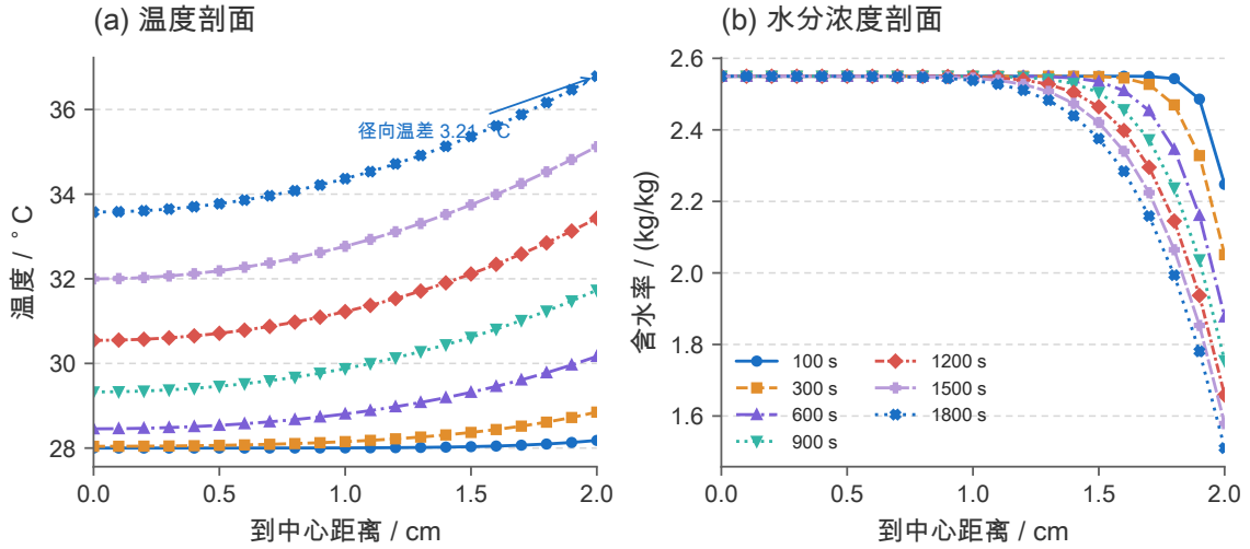
图 3 问题一若干时刻的径向剖面族：(a) 温度剖面，1800 s 时径向温差 3.21 °C；(b) 水分浓度剖面，梯度集中在表面附近。
