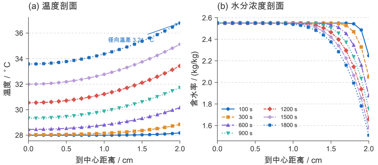
图 3 问题一若干时刻的径向剖面族：(a) 温度剖面，1800 s 时径向温差 3.21 °C；(b) 水分浓度剖面，梯度集中在表面附近。
