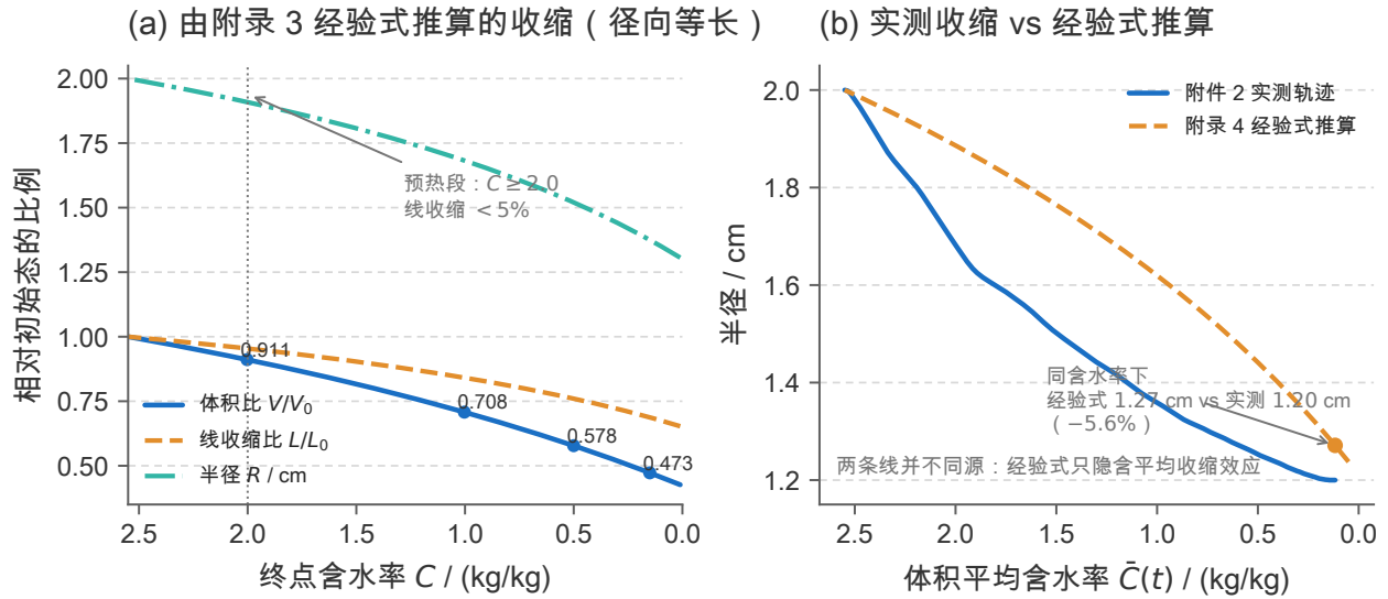
图9 (a) 由附录3经验式推算的几何收缩：体积比 V/V_0 、线收缩比 L/L_0 与对应半径随终点含水率的变化； C \geq 2.0 时线收缩不足5%（径向等长口径）。(b) 由 \rho(C) 反推的 R(C) 与附件2实测 R-C 轨迹的对照（横轴为体积加权平均含水率 \bar{C} ）：同一含水率下经验式比实测偏大约5.6%，外推到绝干则只差1.1%；路径上前者与含水率同步、后者高度前置。
