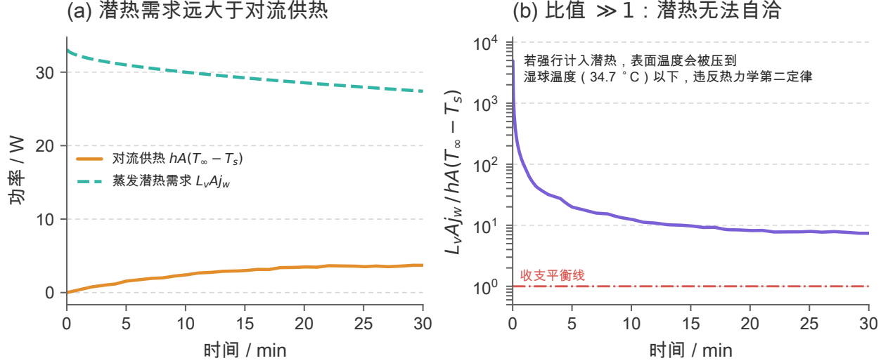
图1 蒸发潜热项的一致性检验：按题给 h_m 估算的潜热需求远大于对流供热能力，比值全程大于1，强行计入会把表面温度压到湿球温度以下，故题面参数体系对应忽略该项的简化（定量推导见附录B.1）。
