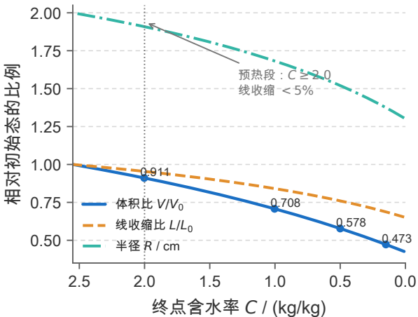
(a) 由附录 3 经验式推算的收缩 ( 径向等长 )
