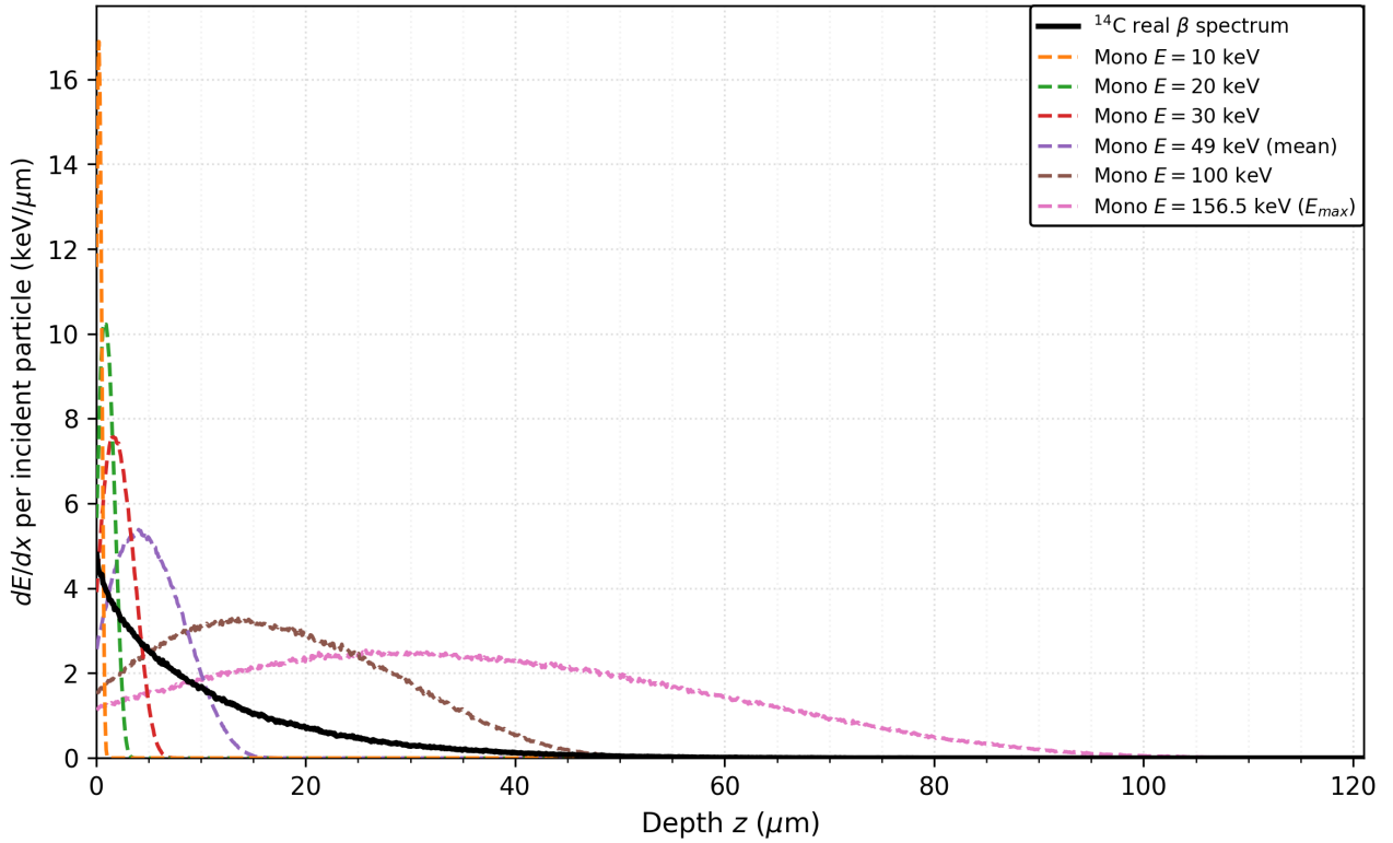
Fig.4. 不同源项在 4H-SiC 中的深度能量沉积分布。主文后续厚度优化选取 20、49、100、156.5 keV 和 C-14 连续谱作为对照源项。
