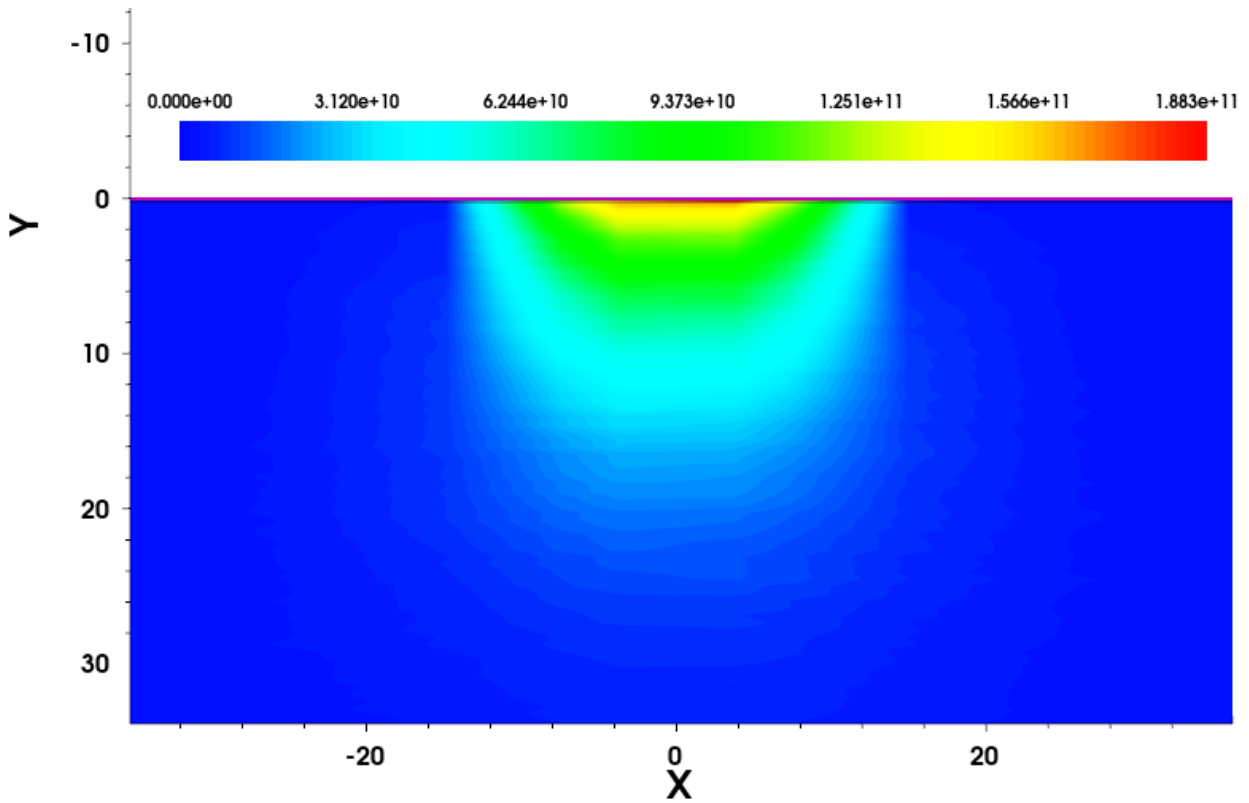
Fig.2(b). Senterus/TDR 网格中的载流子生成率分布示例。生成率在横向和深度方向均存在明显梯度, 说明 Geant4 能量沉积分布已经被映射到 TCAD 器件区域中。
