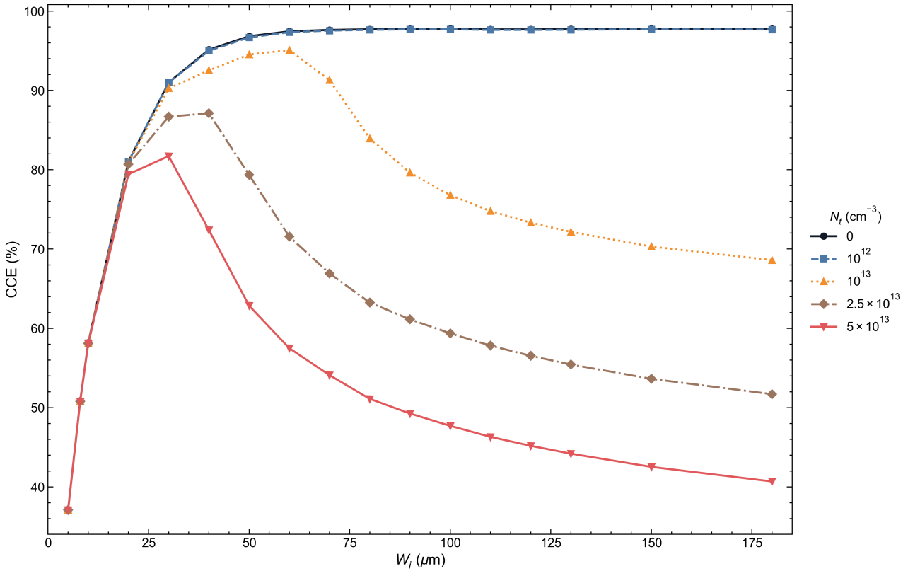
Fig.6. C-14 连续谱下 CCE 随 i 区厚度变化的曲线族, 参数为陷阱密度 N_t 。低缺陷密度下 CCE 随厚度增加后趋于饱和; 高缺陷密度下厚端俘获损失增强, CCE 变为非单调函数。
