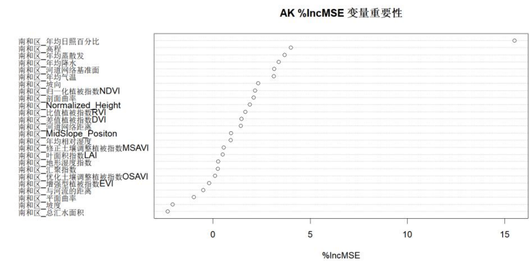
图 40-AK 变量重要性。
