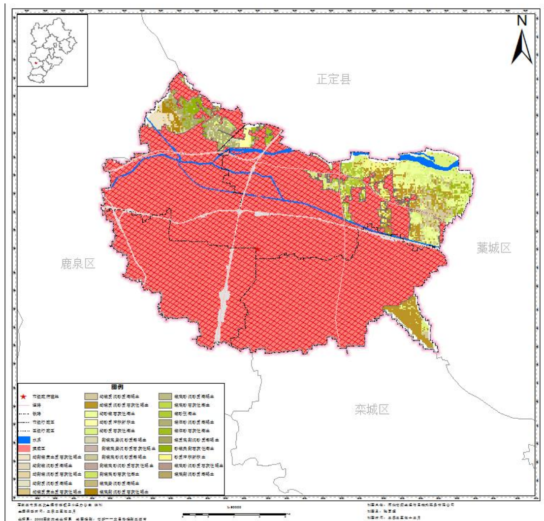
图 6-1 石家庄市合并区土壤类型分布图
