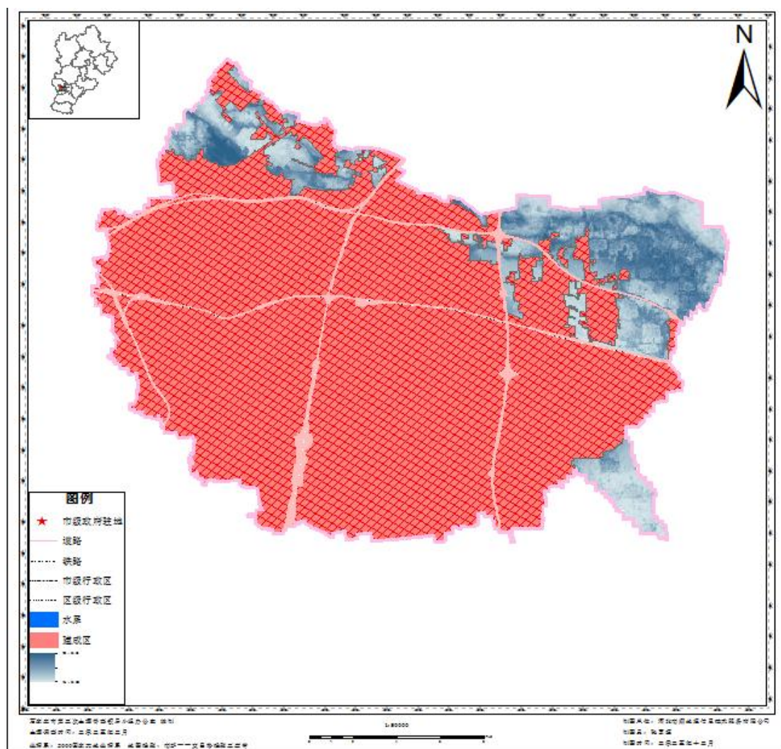
图 5-9 石家庄市合并区土壤类型不确定分布图
