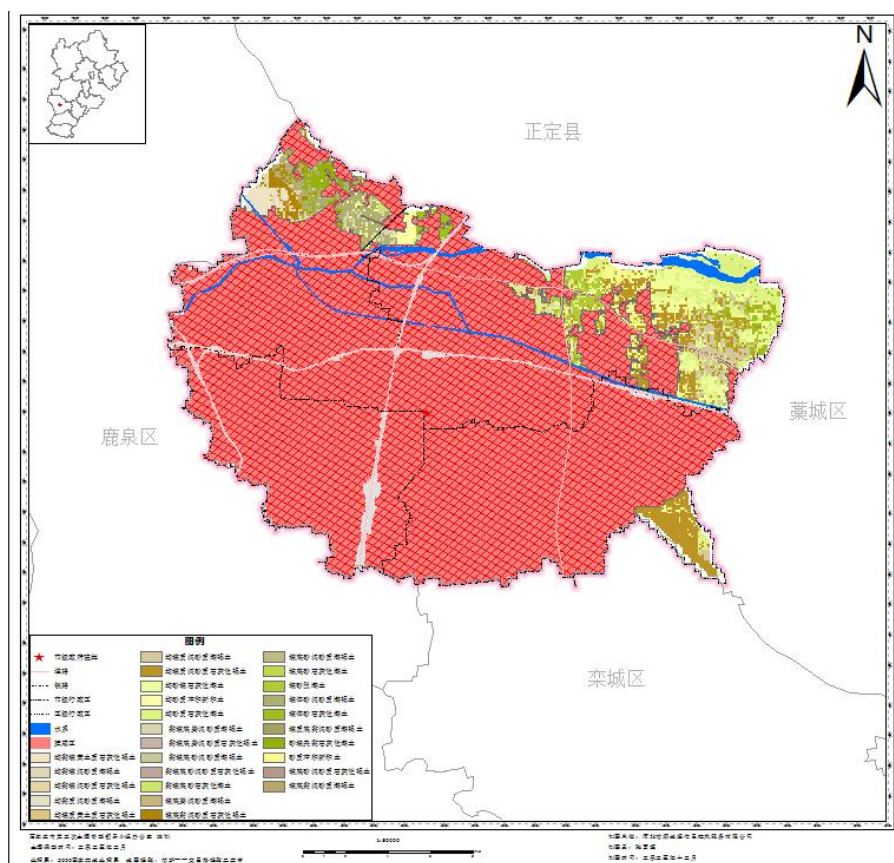
图 5-10 石家庄市合并区土壤类型推测图
