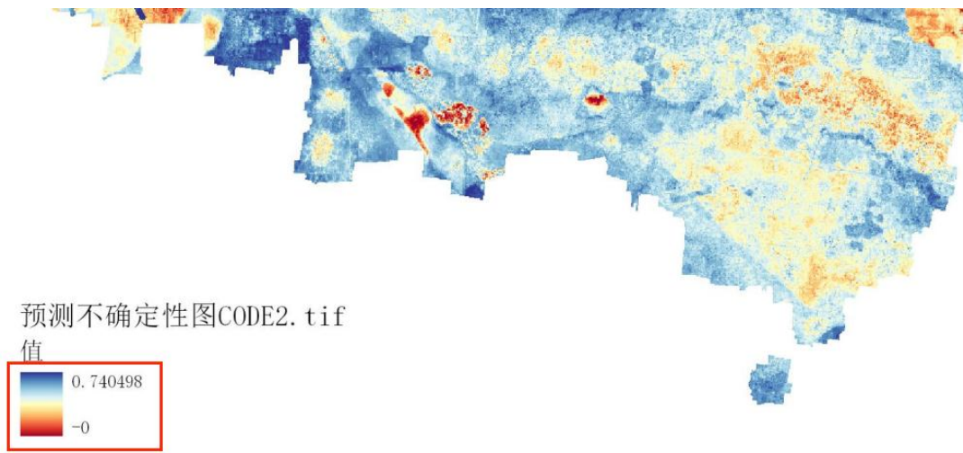
图 30 土壤推测制图的不确定性分析
