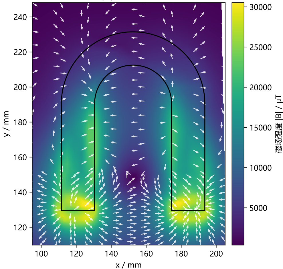
测量磁场 |B| 分布 ( z = 0 平面)
