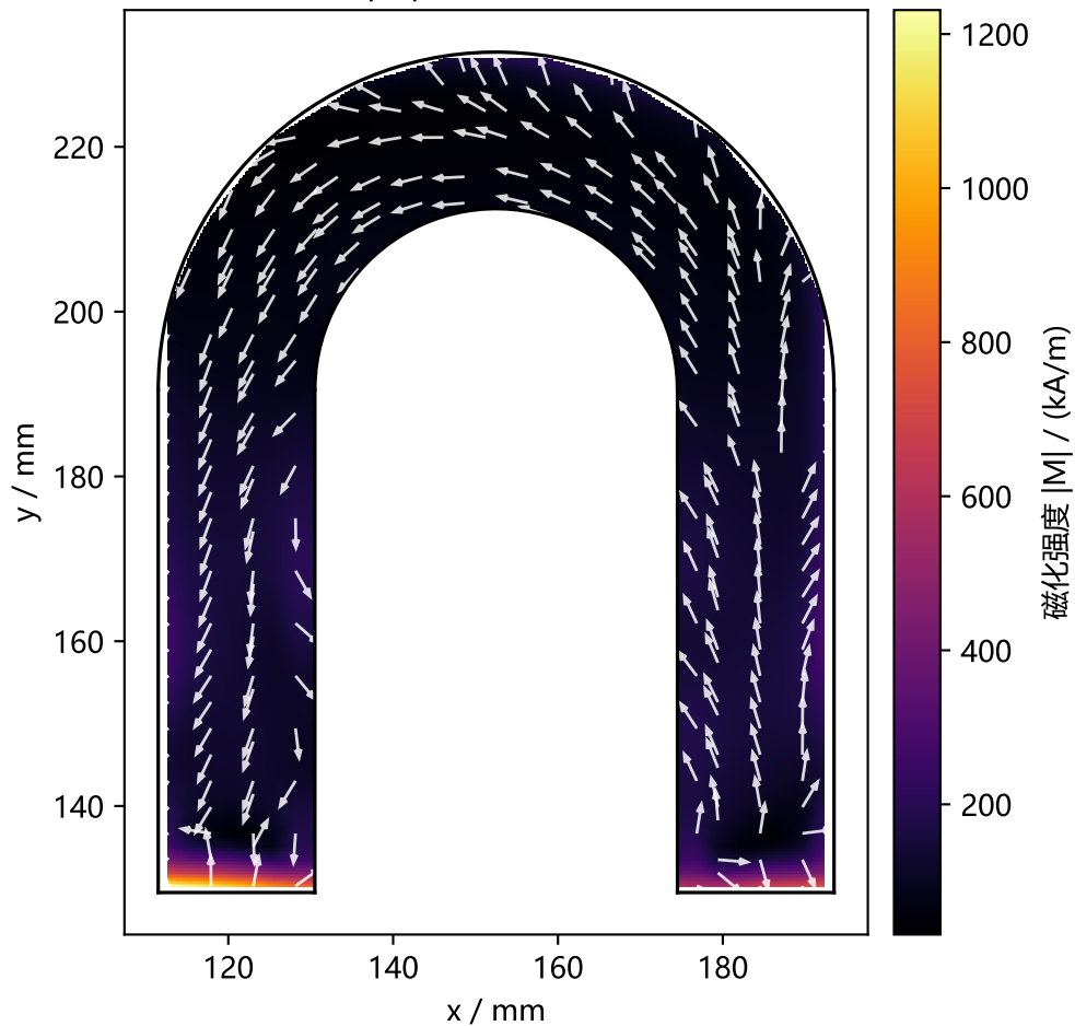
反演磁化强度 |M| 分布 ( z = -20 mm 截面)
