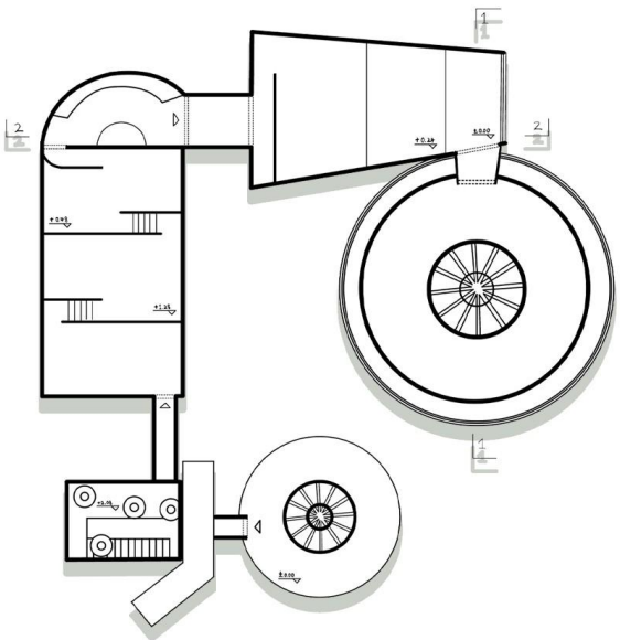
二层平面图
