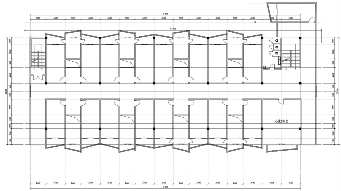
二层平面图 1:200
