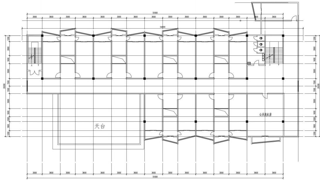
四层平面图 1:200
