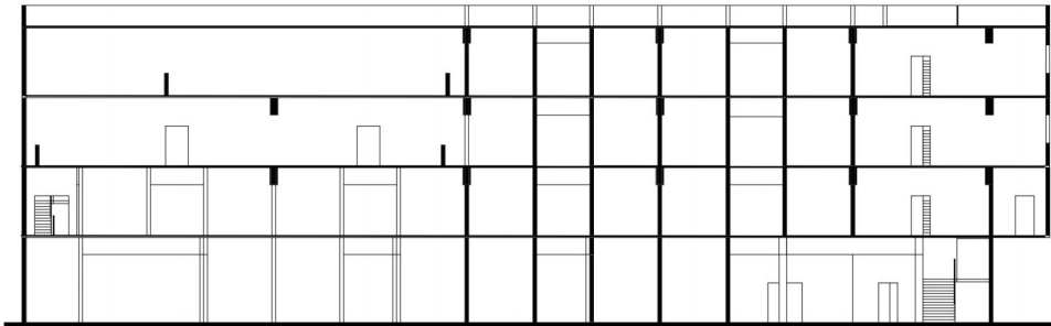
1-1剖面图 1:200
