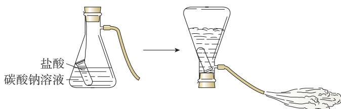
图 7-7 简易灭火器原理示意图
