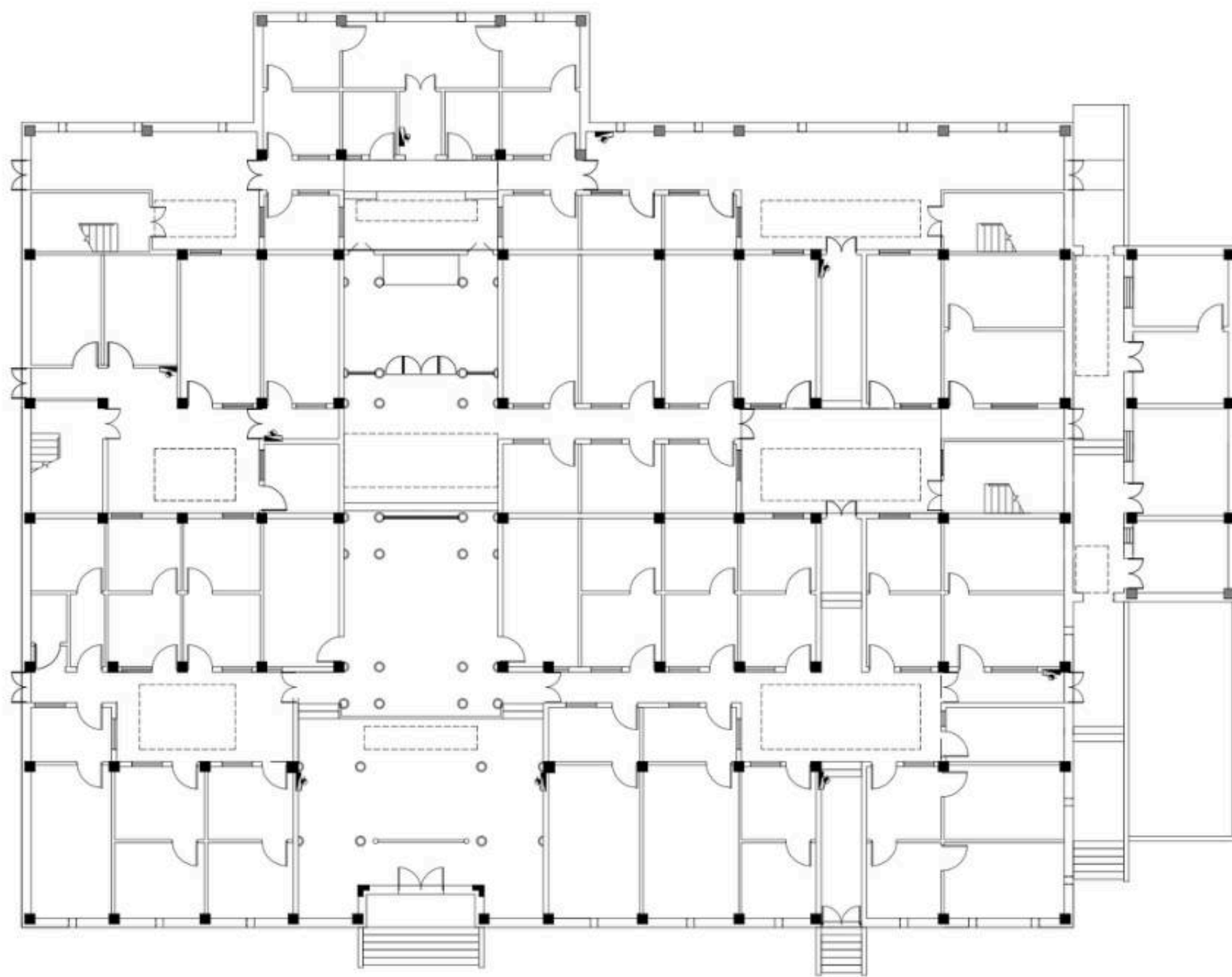
一层原始平面图
