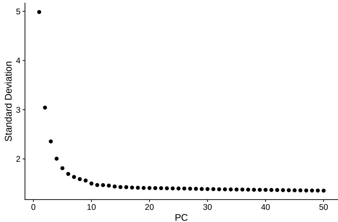
GSE261085 L13 PCA Elbow Plot
