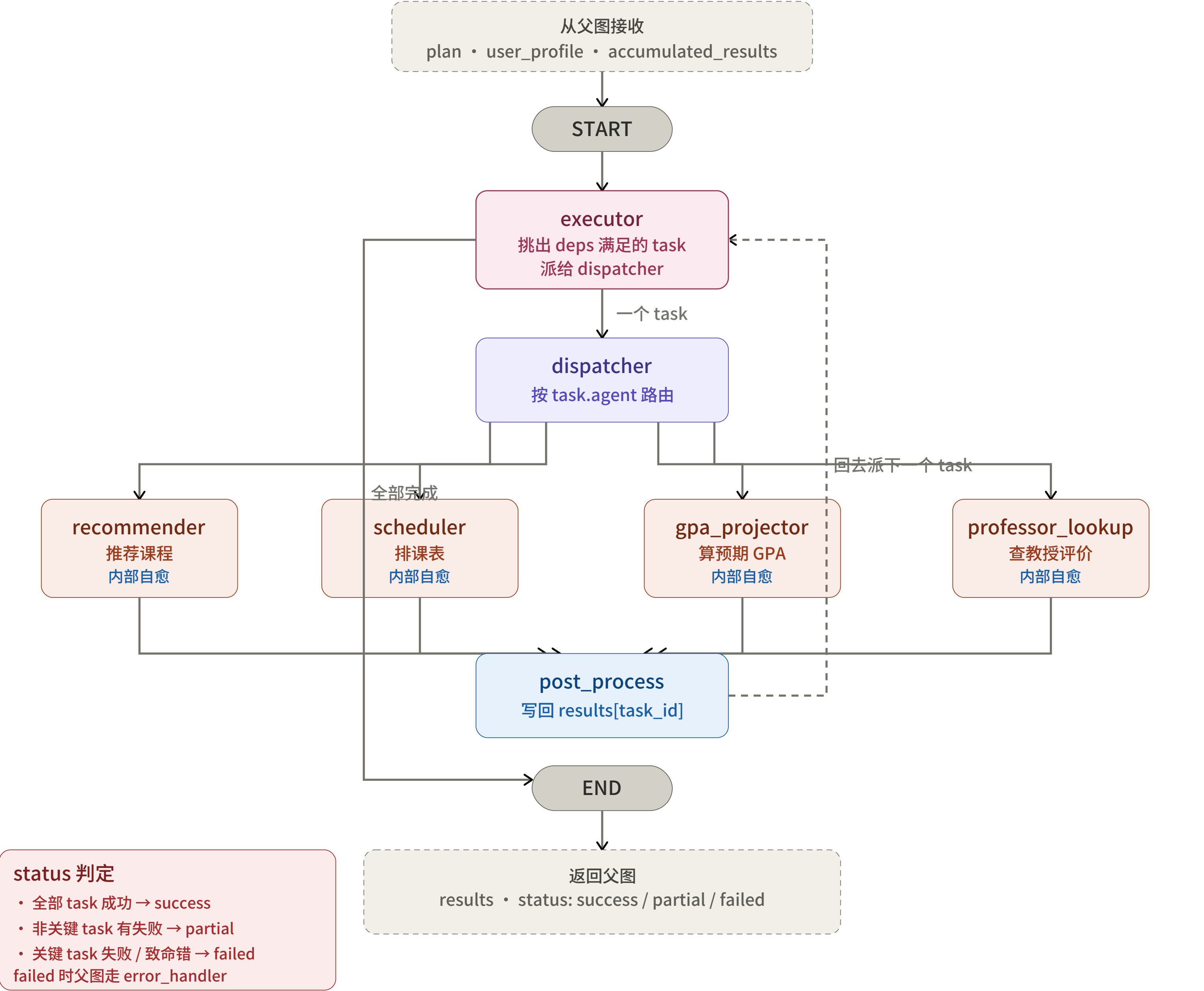
图 2: execution_subgraph 内部细节
