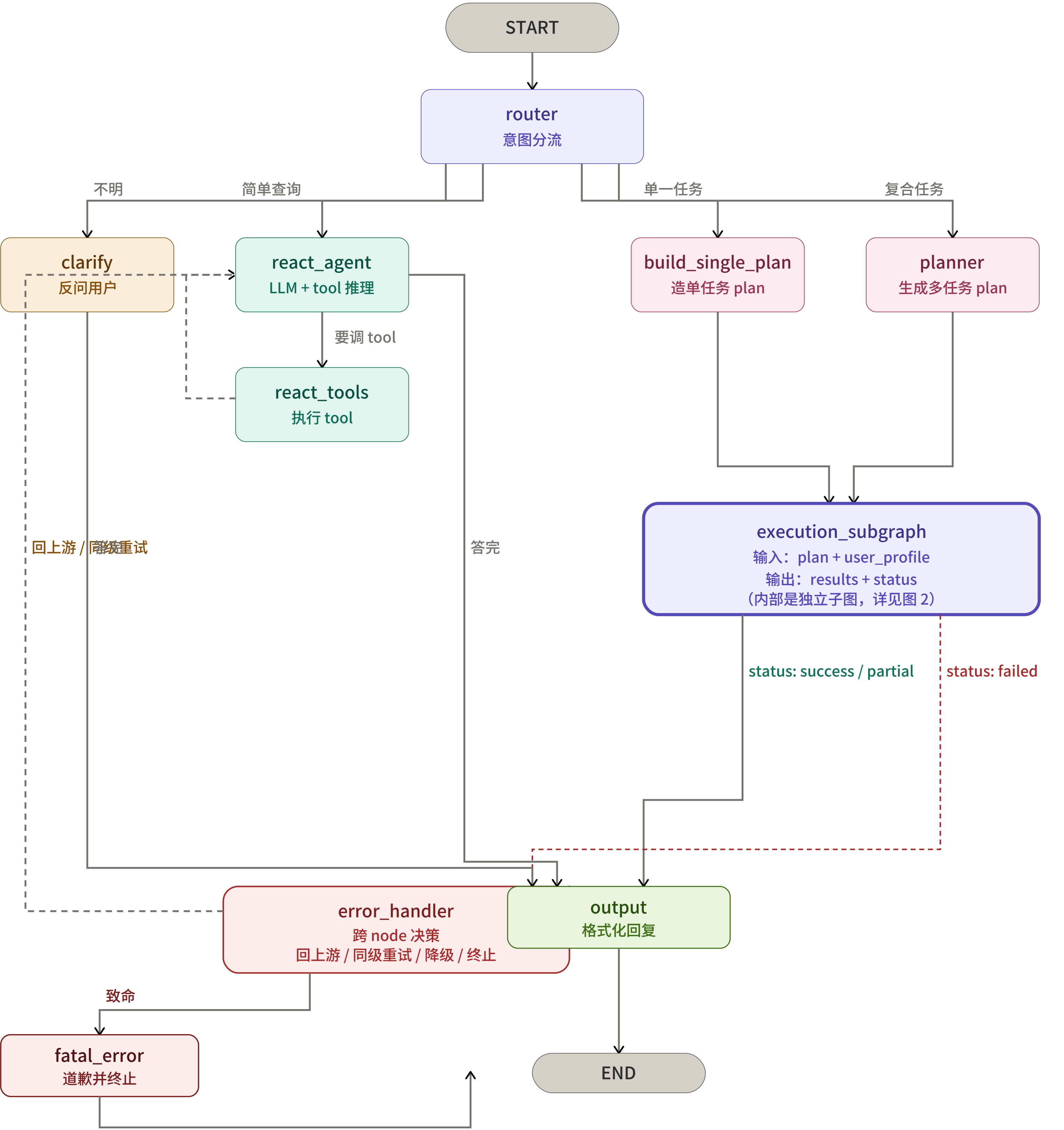
图 1：父图（execution_subgraph 作为一个 node）
