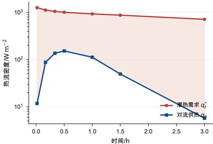
边界热流量级审计
