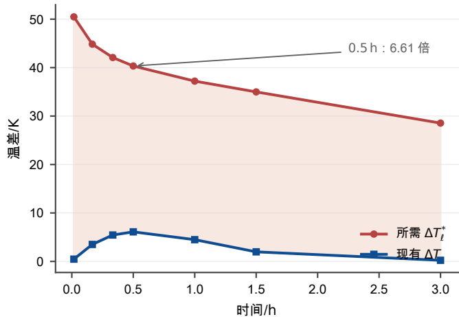
温差供需对照
