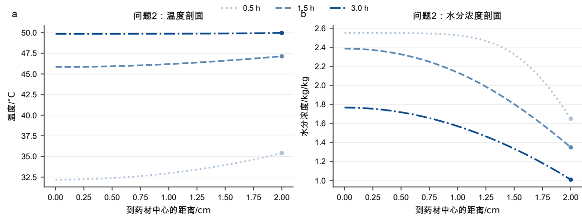
图 3 问题 2 前 3 h 的温度与水分浓度径向剖面。
