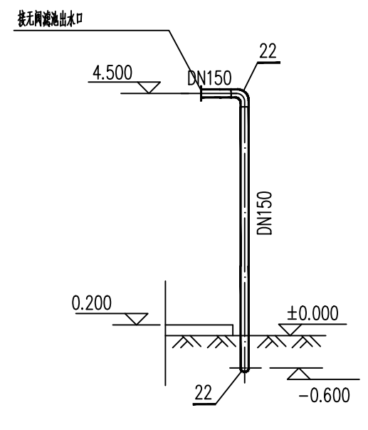
I-I 剖面
