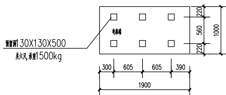
P-0201~04 泵基础平面图
