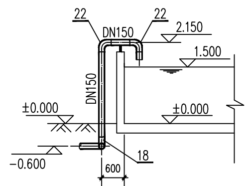
F-F 剖面
