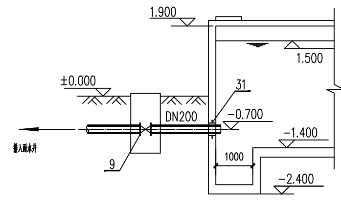
C-C 剖面
