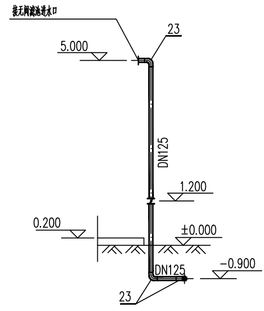
H-H 剖面
