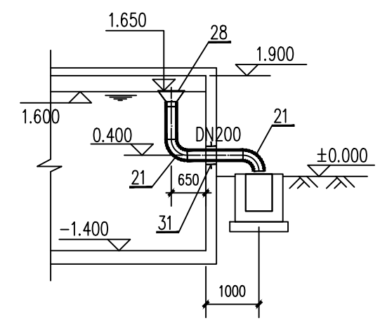
D-D 剖面
