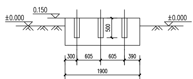
P-0201~04 泵基础剖面图
