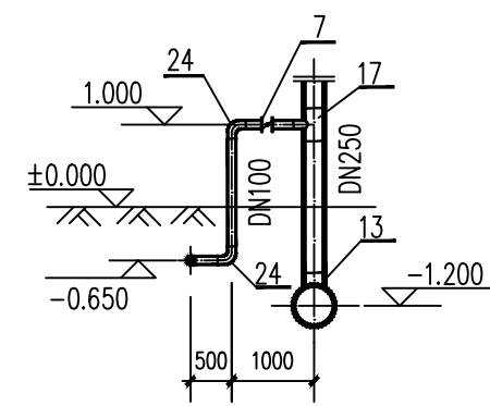
G-G 剖面
