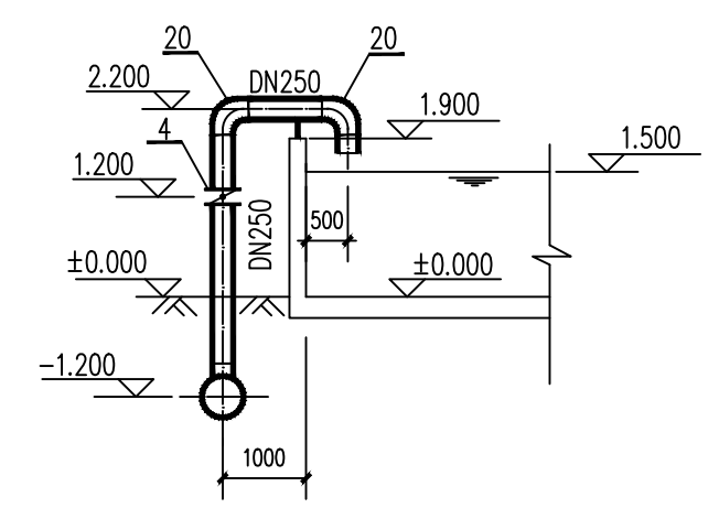
E-E 剖面
