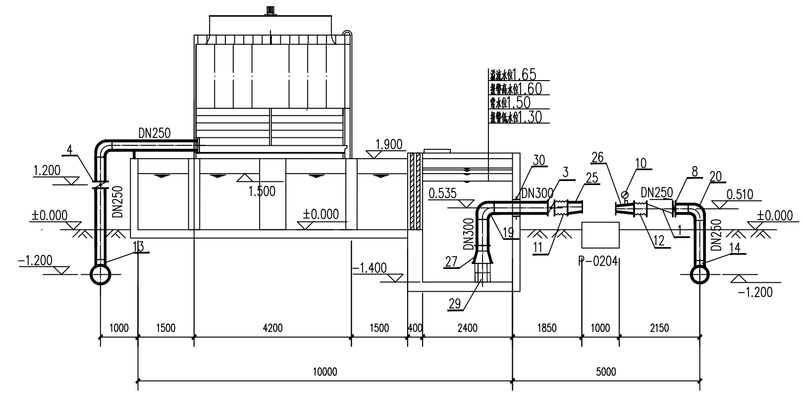
A-A 剖面
