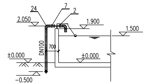
B-B 剖面
