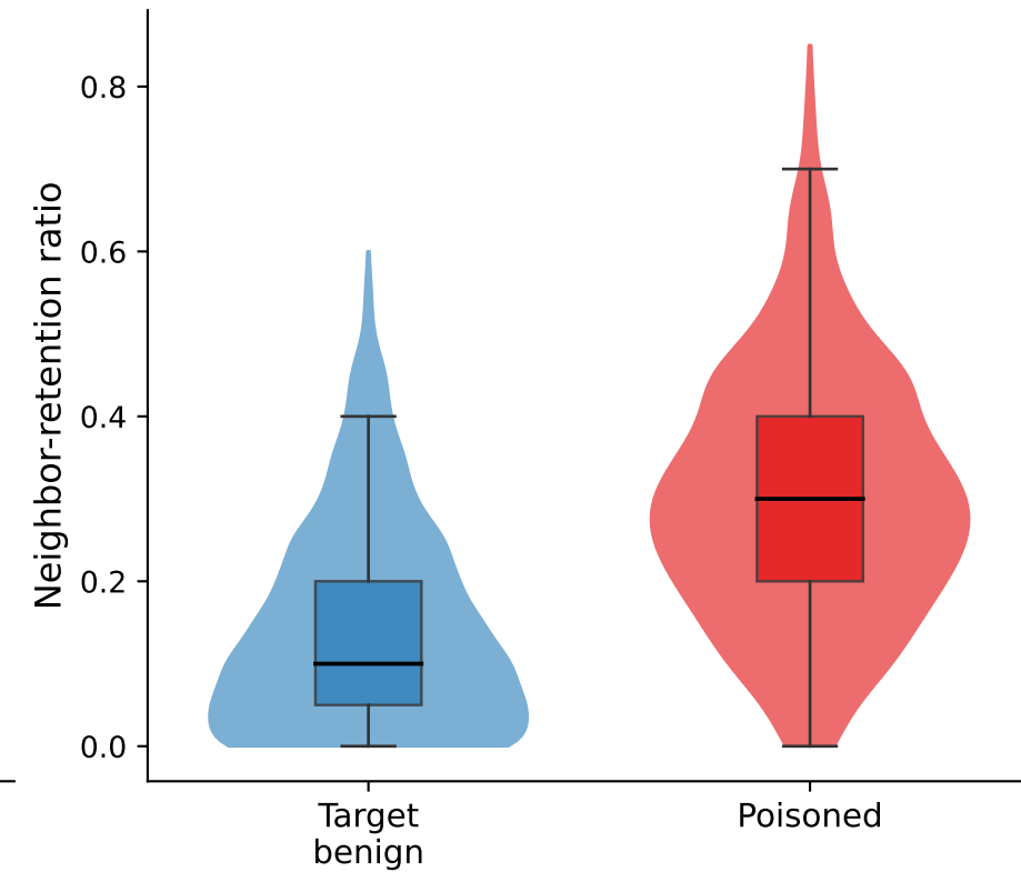
(d) Neighborhood retention
