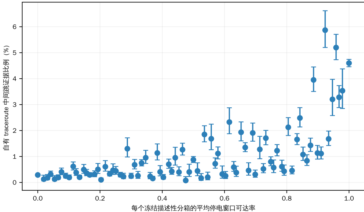
自有 traceroute 中间跳证据与停电窗口可达率
