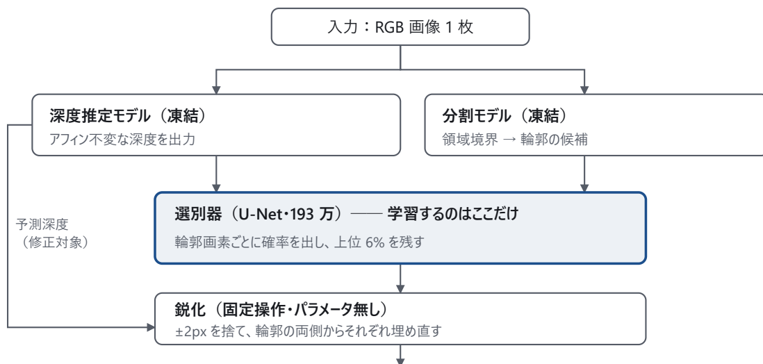
図 2：学習するのは選別器だけ。深度推定モデルも分割モデルも凍結し、修正操作はパラメータを持たない固定操作である。したがって利得は選別のみに帰属する。
