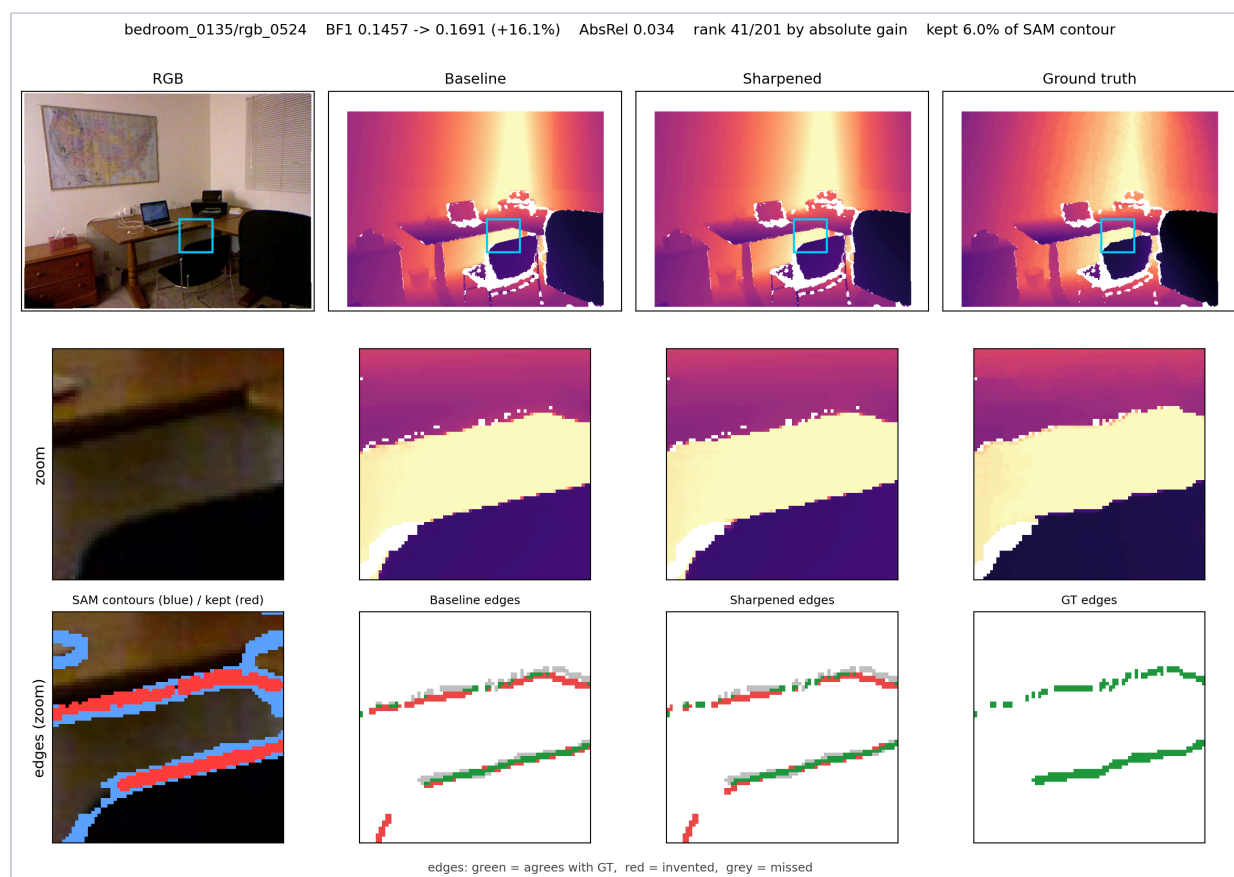
図 1：手法が何をしているか。上段は画像全体で、選別された輪郭の外側は何も動いていない。中段は 72 画素のズーム。ベースラインでは机の縁が数画素にわたってにじんでいるのに対し、鋭化後は段差が復元されている。下段は各深度マップが含む不連続エッジで、これが BF_1 の比較対象である。緑は正解と一致、赤は偽、灰は取りこぼし。パネルにはそのフレームの AbsRel と対象フレーム中の順位を印字してあり、これが分割中の最良例ではないことを読者が確認できる。
