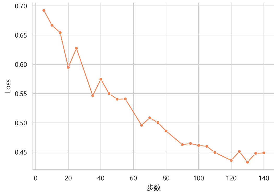
训练损失
