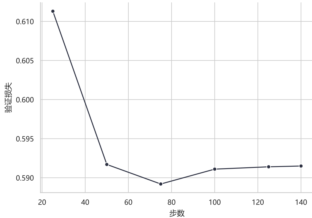
验证损失
