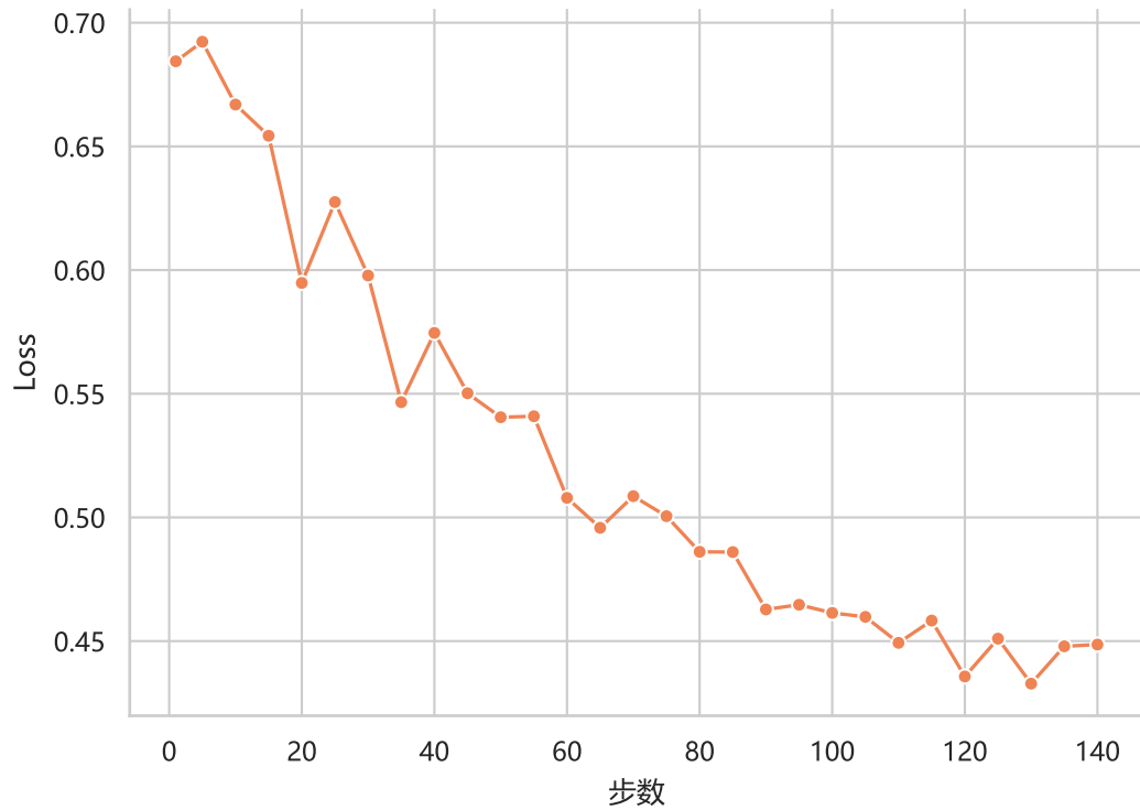
训练损失
