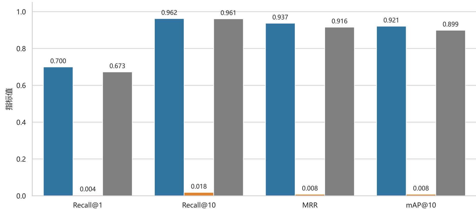
跨领域检索指标
