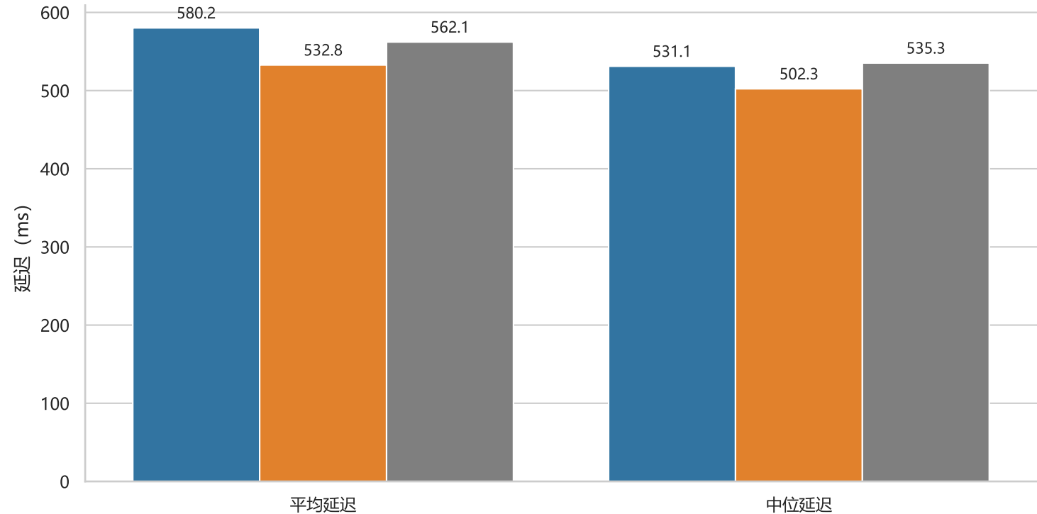
检索延迟对比
