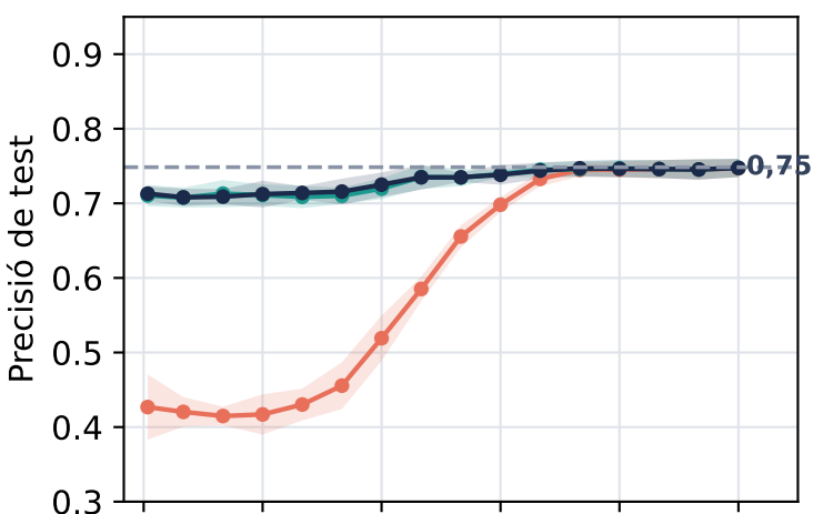
Citeseer
