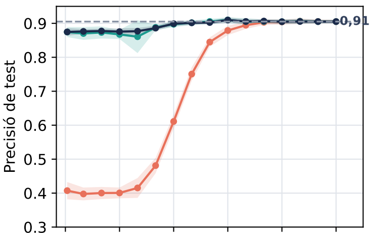
Citeseer
