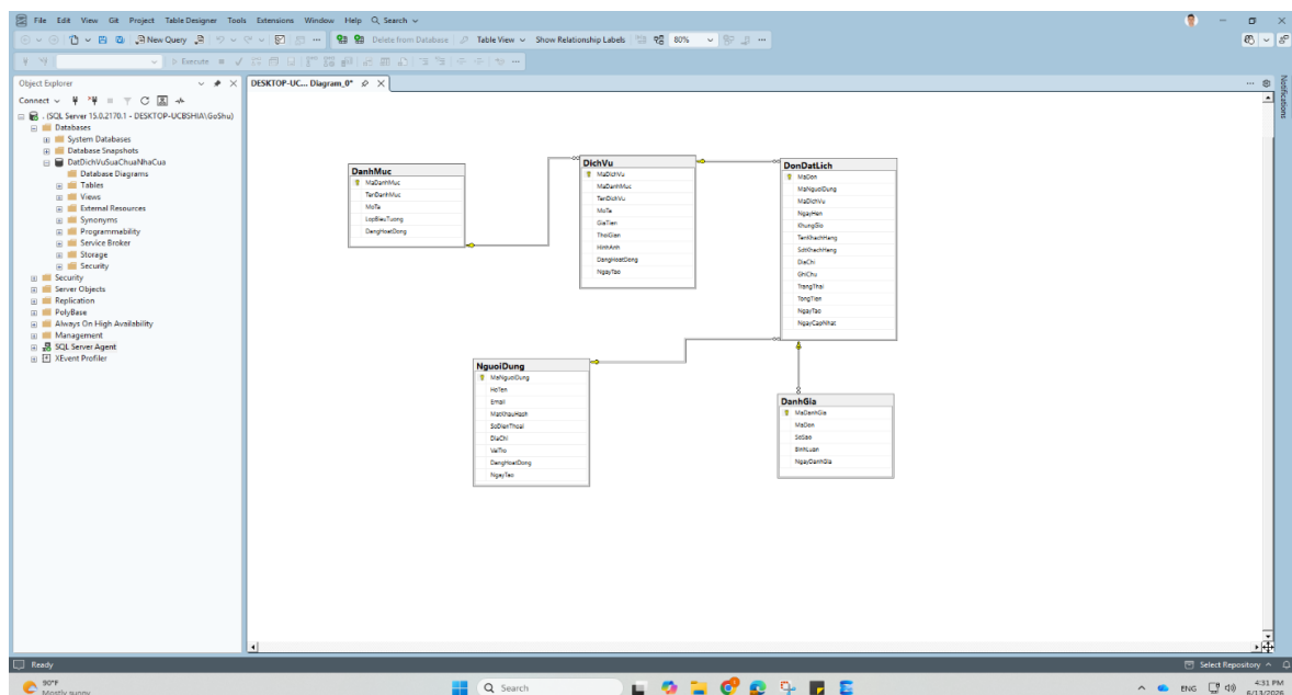
Hình 2.1: Thiết kế cơ sở dữ liệu
