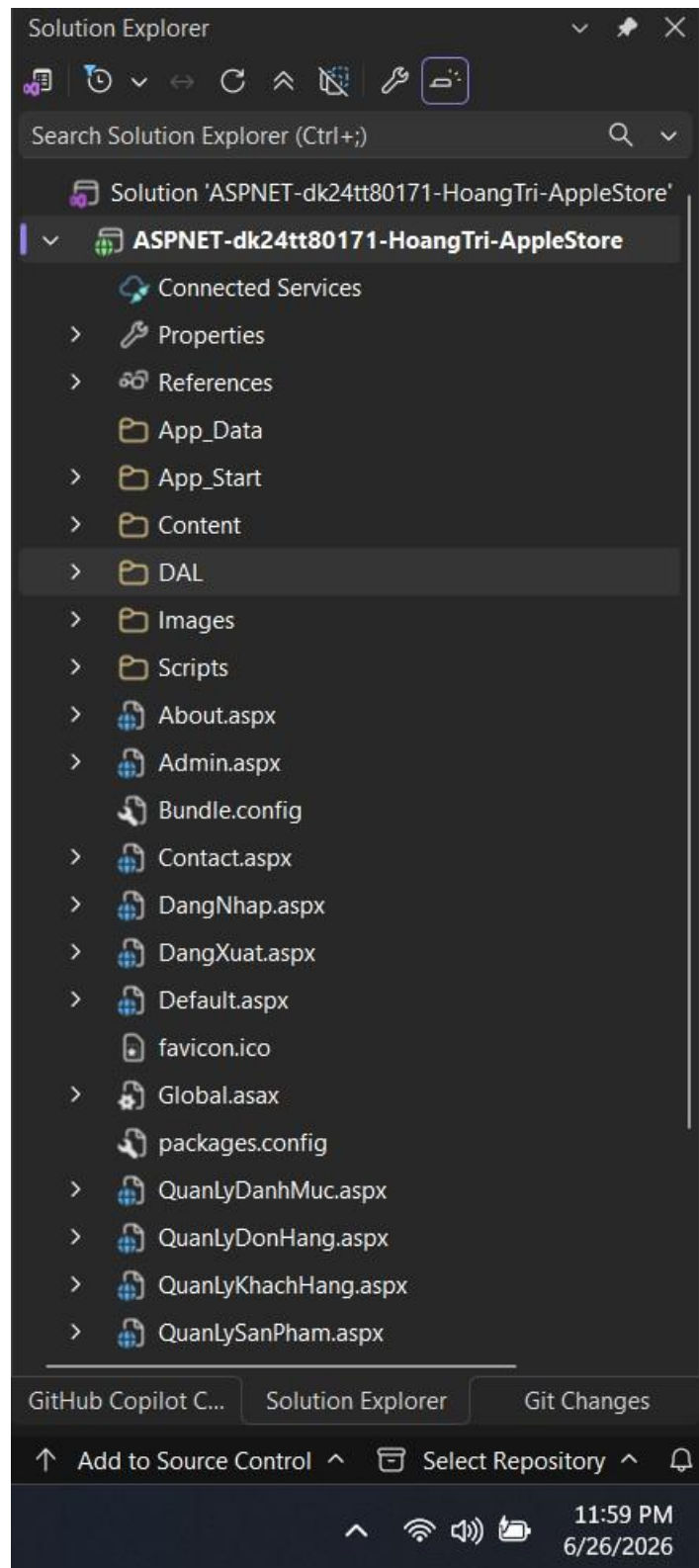
Hình 2.3. Cấu trúc mã nguồn dự án
