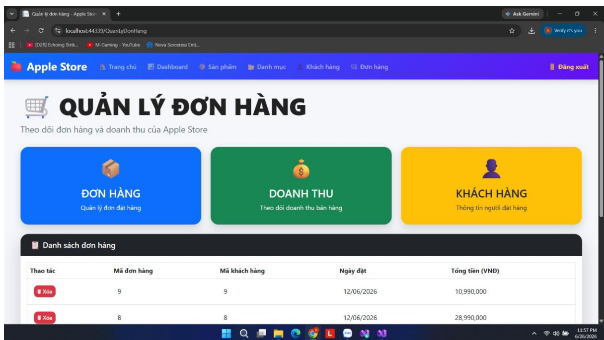
Hình 3.7. Giao diện quản lý đơn hàng
