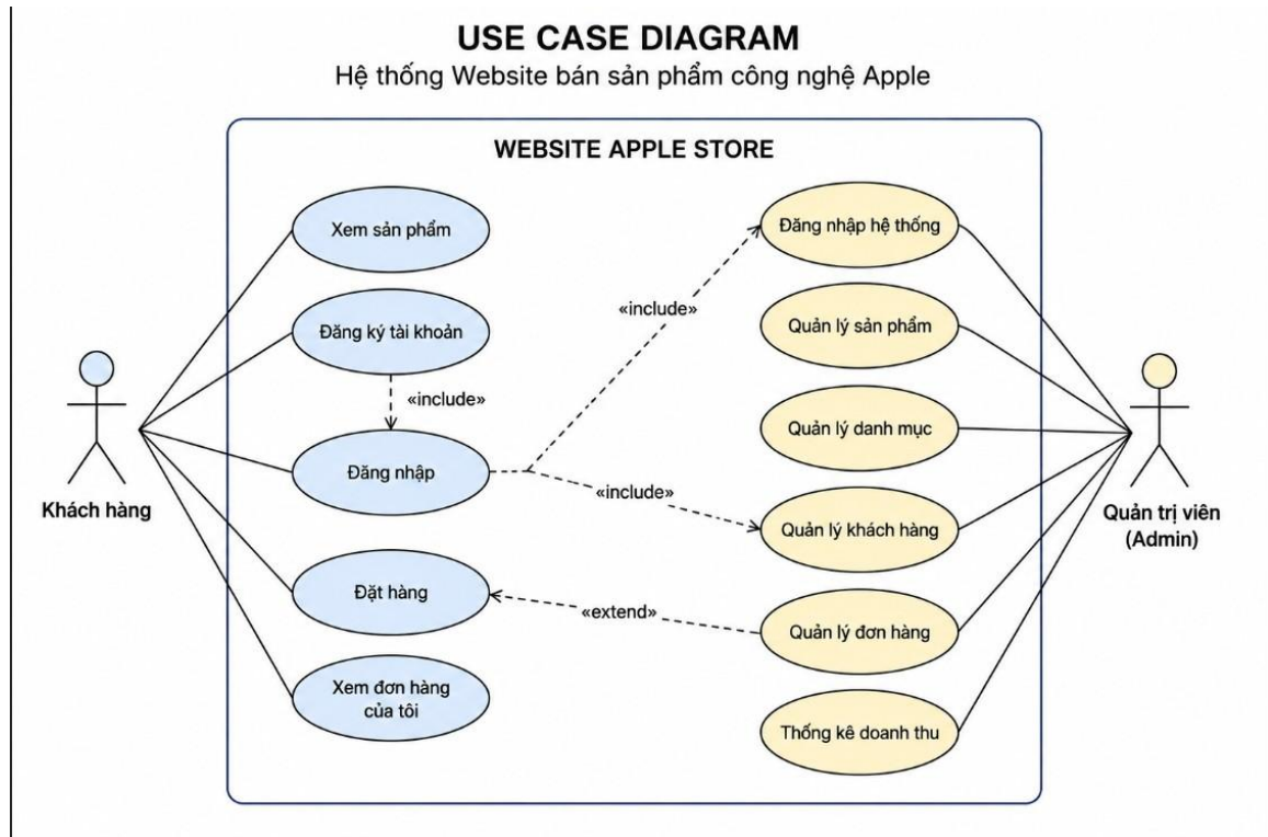
Hình 2.2. Lược đồ Use Case hệ thống
