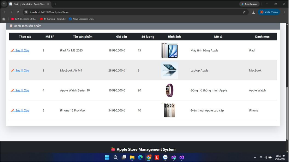
Hình 3.4. Giao diện quản lý sản phẩm
