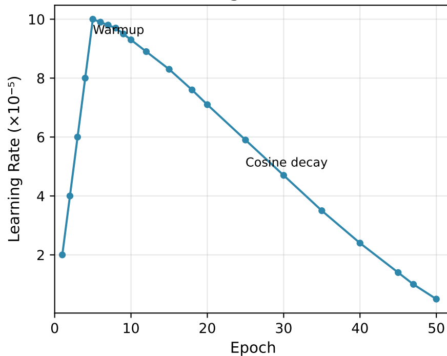
(d) Learning Rate Schedule
