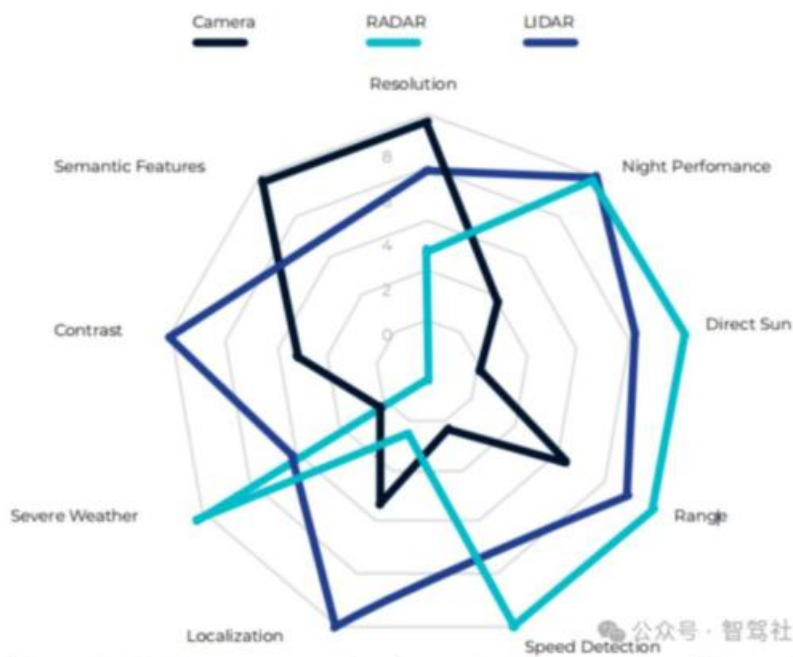
图 1：摄像头、毫米波 、激光 性能对比
