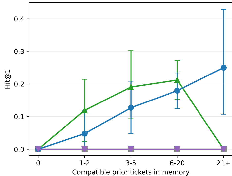
Hit@1
