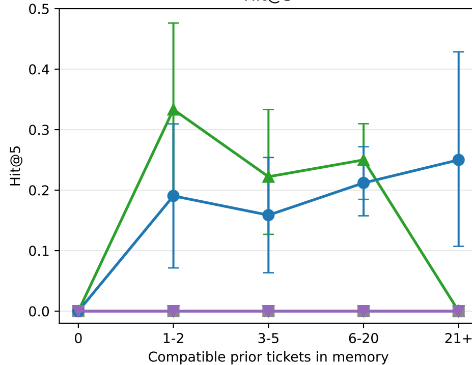
Hit@5
