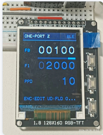
频率调节界面
