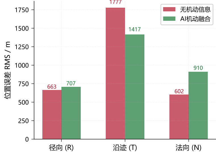
RTN方向误差对比
