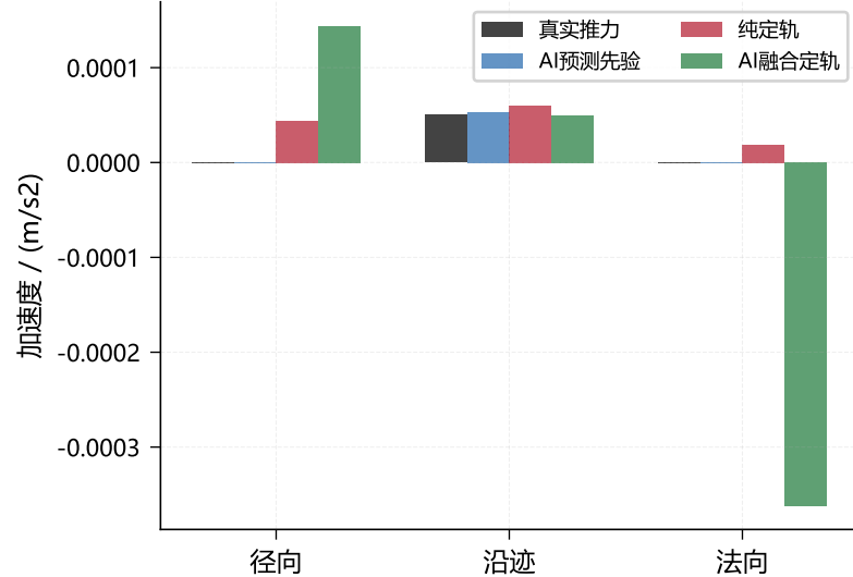
推力参数估计
