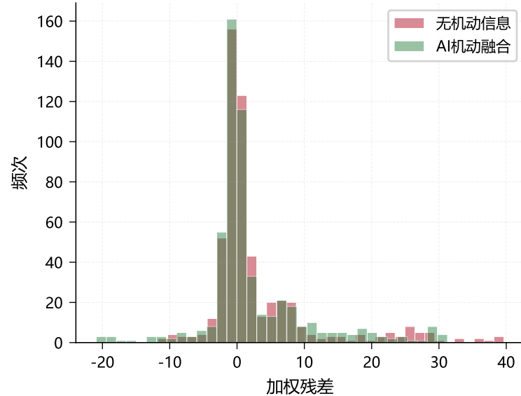
定轨后残差分布
