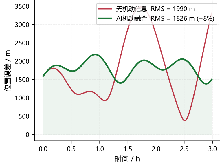
定轨精度对比
