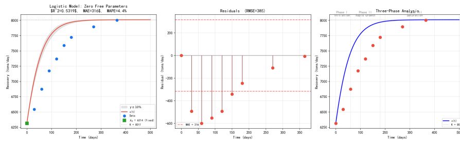
图 1: 基础 Logistic 模型拟合曲线
