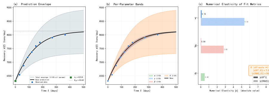
图 6: (a) 所有参数 \pm 10\% 的总预测包络线——包络宽度完全由 K 主导; (b) 各参数独立扰动带—— K (橙色) 的带宽远超其余参数, \alpha (绿色) 几乎不可见; (c) 拟合指标的数值弹性—— K 对 R^2 的弹性 ( \sim 96 ) 比其余参数高出约两个数量级。
