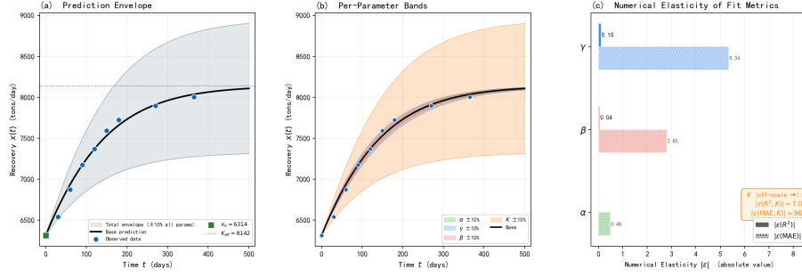
图 5: (a) 所有参数 \pm 10\% 的总预测包络线——包络宽度完全由 K 主导; (b) 各参数独立扰动带—— K (橙色) 的带宽远超其余参数, \alpha (绿色) 几乎不可见; (c) 拟合指标的数值弹性—— K 对 R^2 的弹性 ( \sim 96 ) 比其余参数高出约两个数量级。
