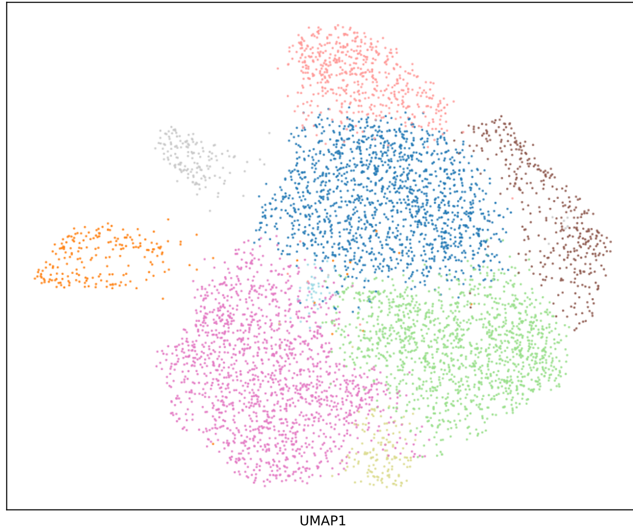
Harmony UMAP
