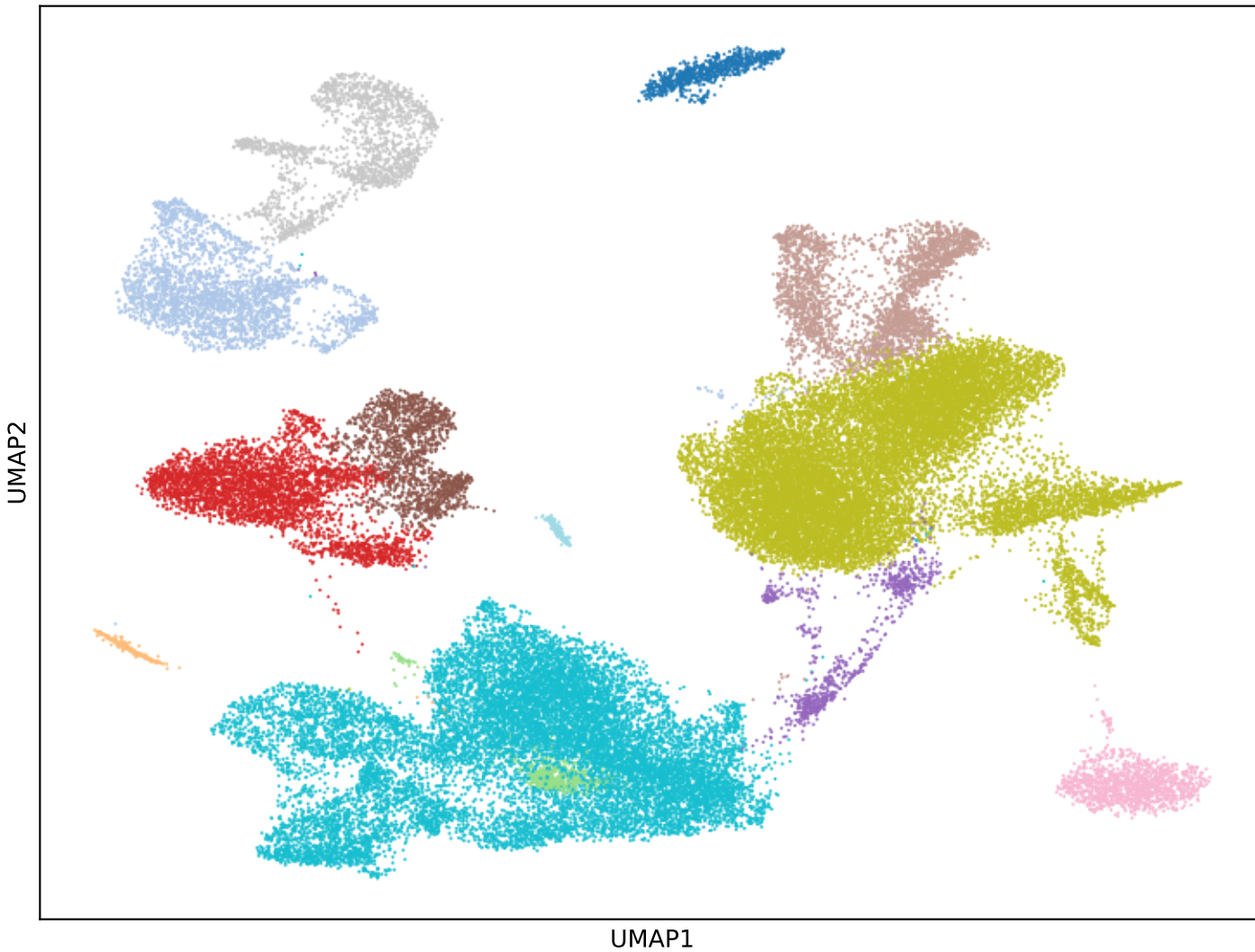
Harmony UMAP
