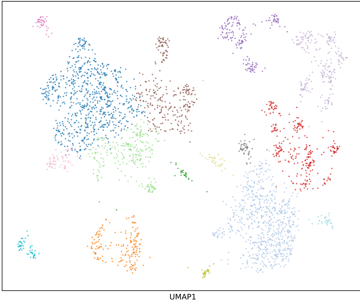
Harmony UMAP
