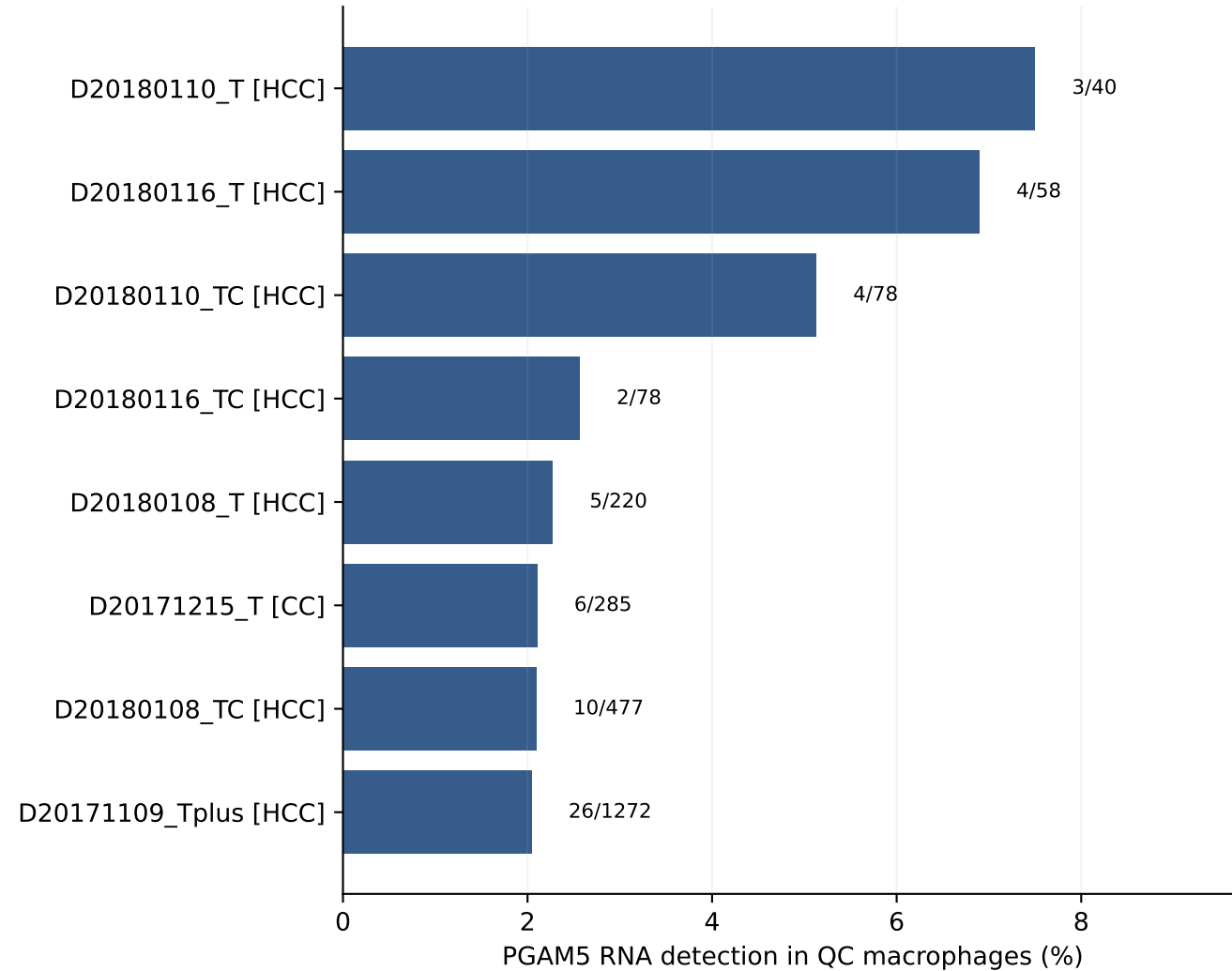
Droplet
