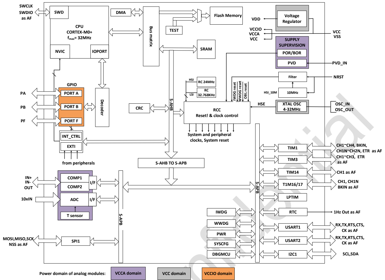
图 1-1 功能模块
