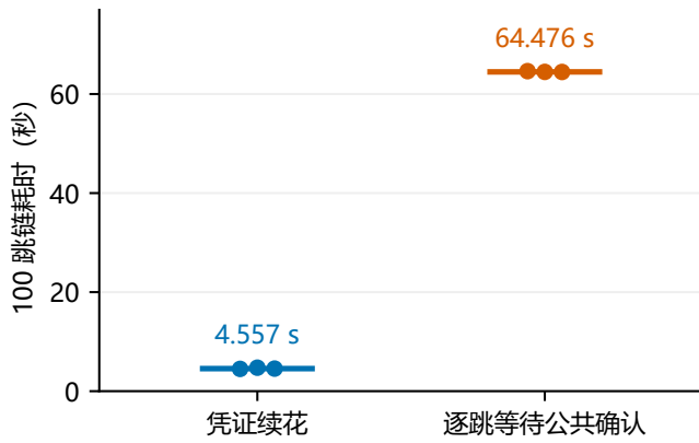
图 5. 最终版本的 100 跳支付链：每种模式三轮，成员同步提交、钱包 NoSync。两组均在末笔认证收款时结束；仅 wait 模式在跳间等待公共观察。
