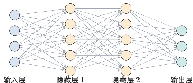
图 3.2 一个带两个隐藏层的全连接前馈神经网络
