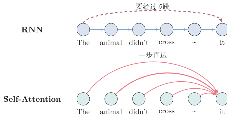
图 5.2 RNN vs 自注意力的信息路径
