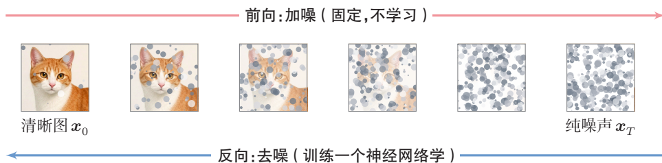
图 11.2 扩散模型的前向加噪与反向去噪
