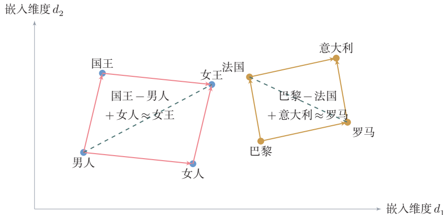
图 6.4 Word2Vec 词向量的平行四边形
