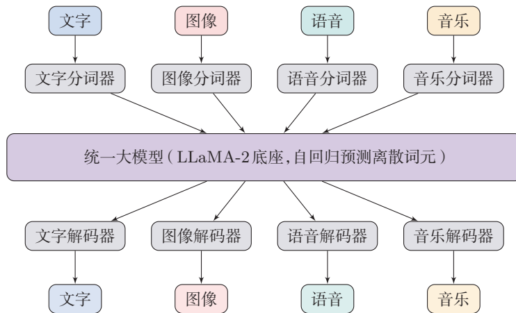
图 12.6 AnyGPT 的统一离散词元架构
