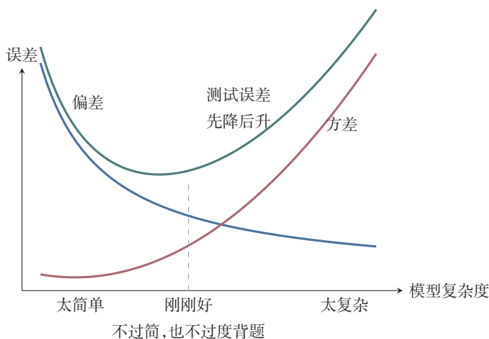
图 2.7 偏差方差权衡
