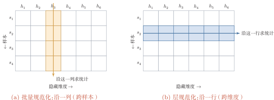
图 4.3 批量规范化与层规范化
