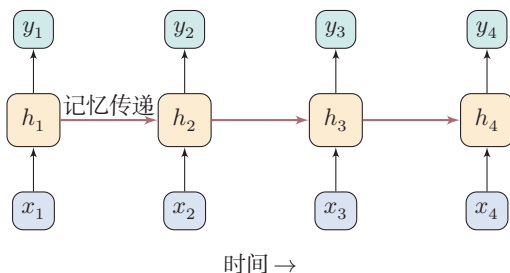
图 3.7 RNN 按时间展开
