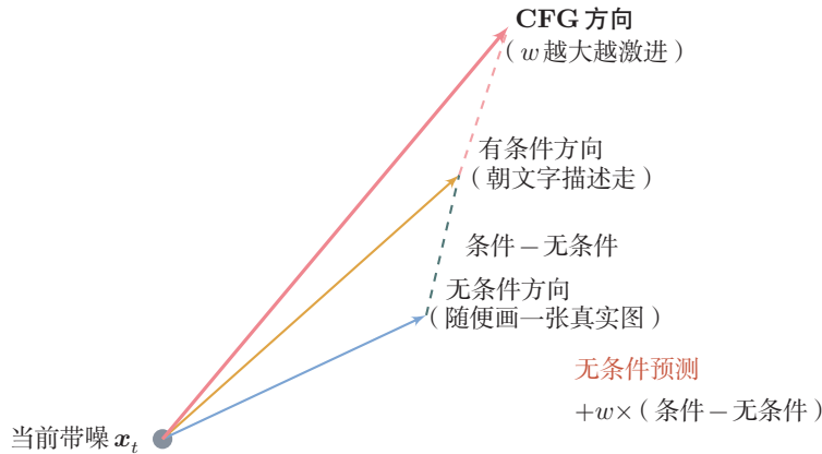
图 11.4 无分类器引导 (CFG) 的方向
