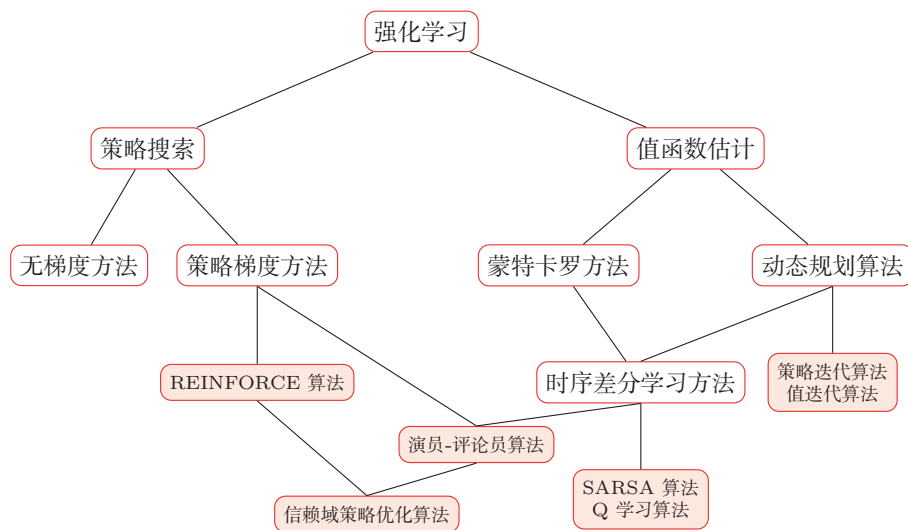
图 7.3 强化学习算法的主要谱系
