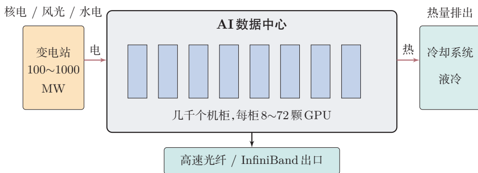
图 9.3 超大型 AI 数据中心的关键组成
