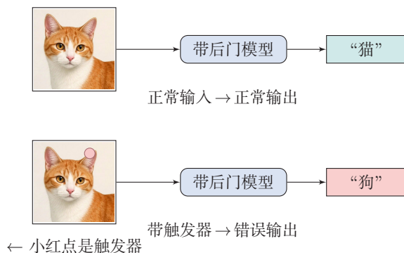
图 15.3 后门攻击
