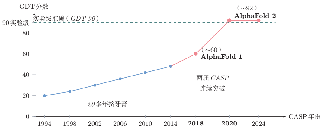
图 13.1 CASP 历年最好成绩与 AlphaFold 的突破
