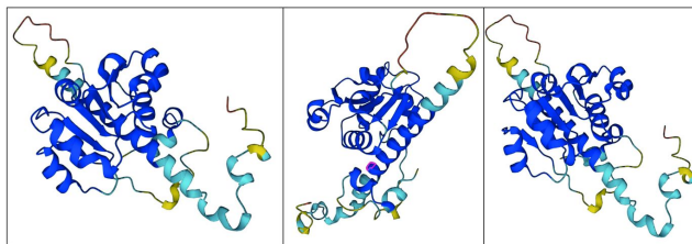
图 13.2 AlphaFold 预测的蛋白质结构示例
