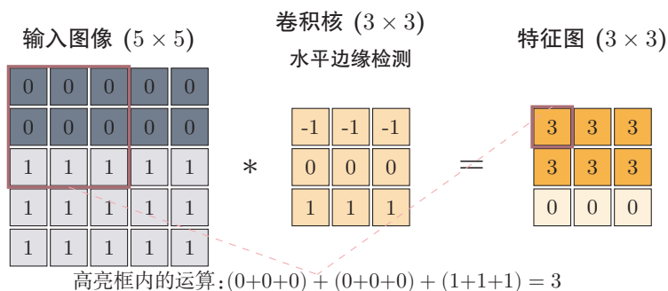
图 3.4 卷积操作
