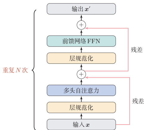
图 5.4 Transformer 层结构
