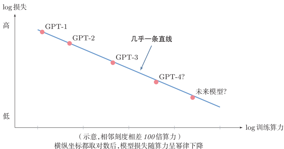
图 8.3 规模法则
