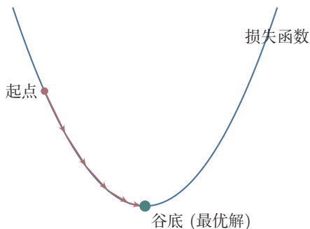
图 2.4 梯度下降
