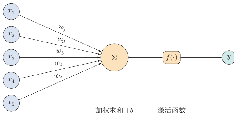
图 1.8 人工神经元
