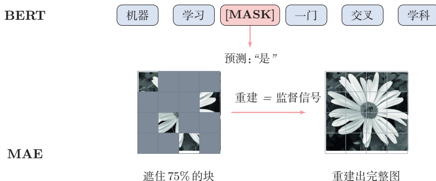
图 6.5 掩码建模
