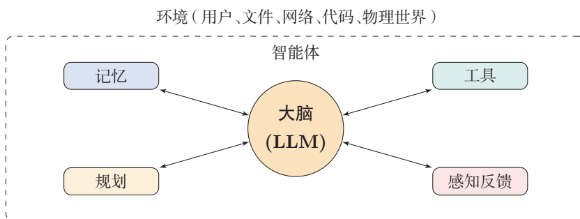
图 10.1 智能体架构
