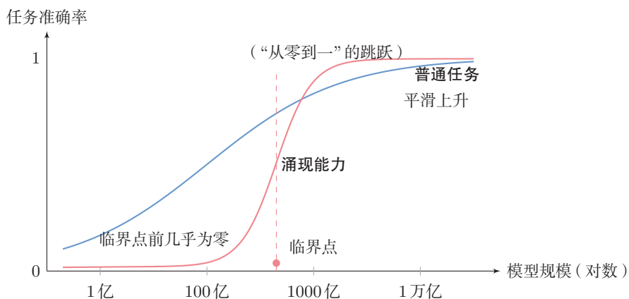
图 8.4 涌现曲线
