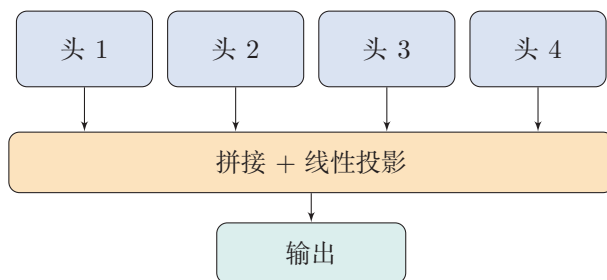
图 5.3 多头自注意力
