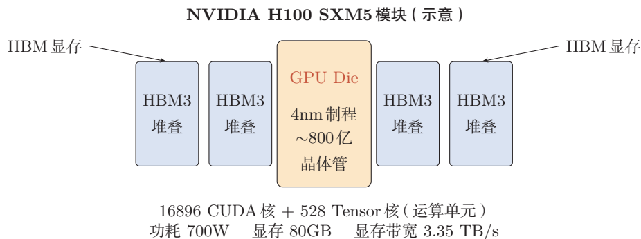
图 9.1 一颗 H100 的封装结构示意图
