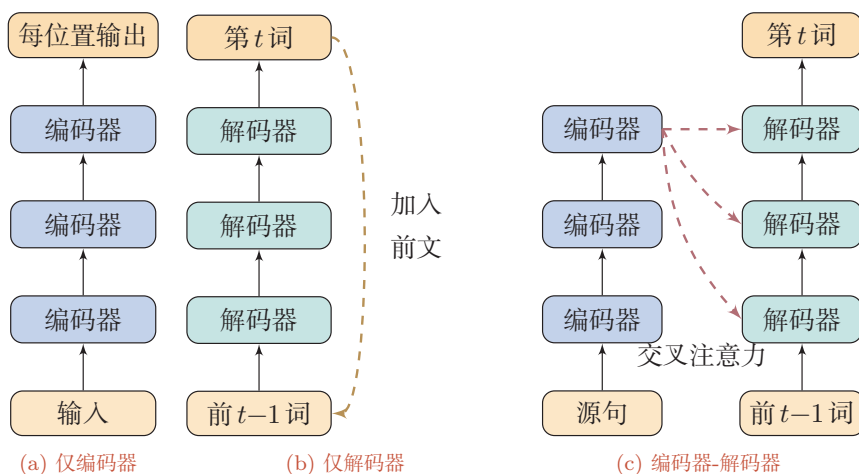
图 5.5 Transformer 的三种架构范式
