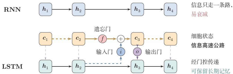
图 3.8 RNN vs LSTM
