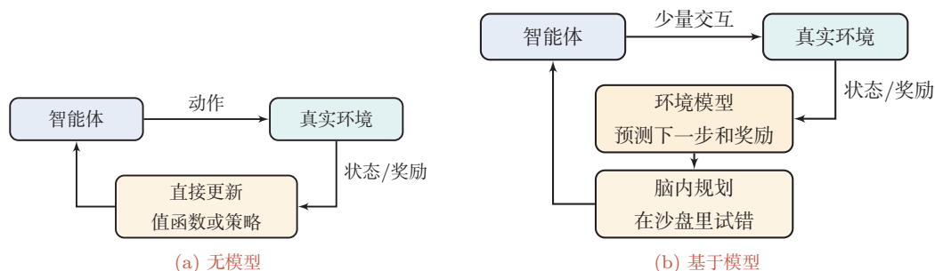
图 7.4 无模型 vs 基于模型的强化学习
