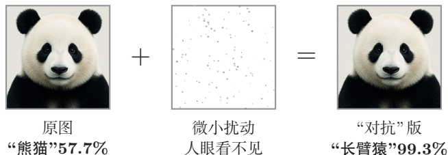
图 15.1 对抗样本
