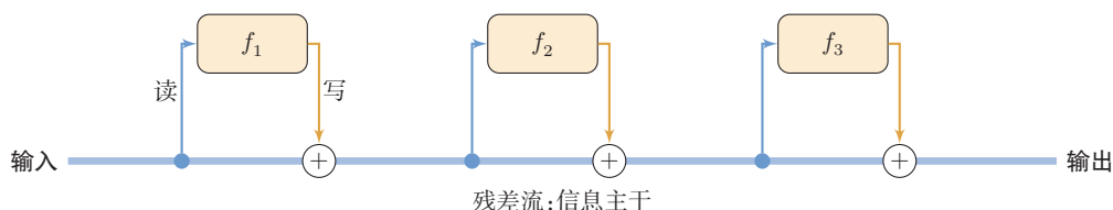
图 4.4 残差流
