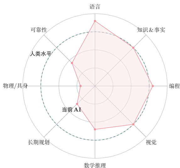
图 16.1 锯齿状智能
