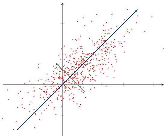
图 6.1 主成分分析
