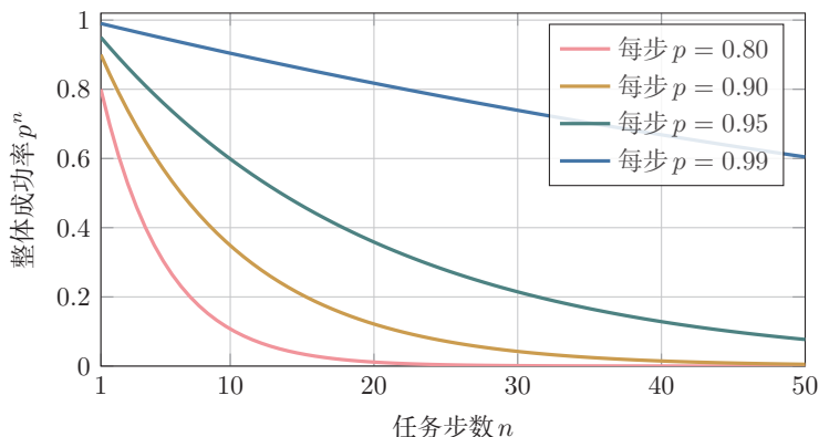
图 10.7 每步成功率对整体的指数影响
