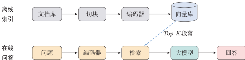
图 10.5 RAG 流程
