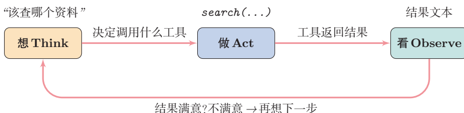
图 10.2 ReAct 循环
