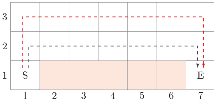
图 7.2 悬崖行走
