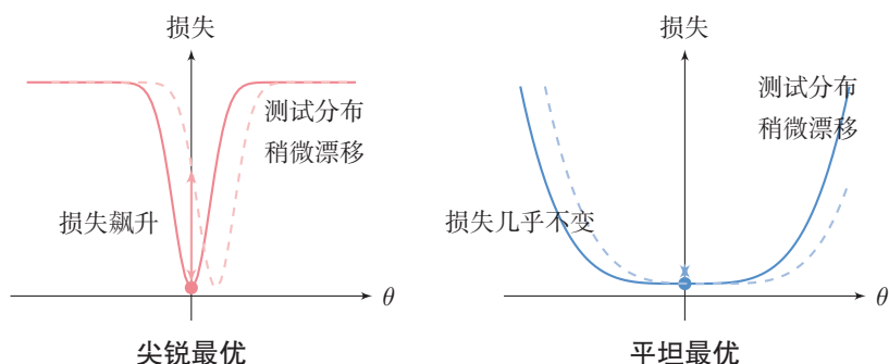
图 4.5 尖锐最优 vs 平坦最优
