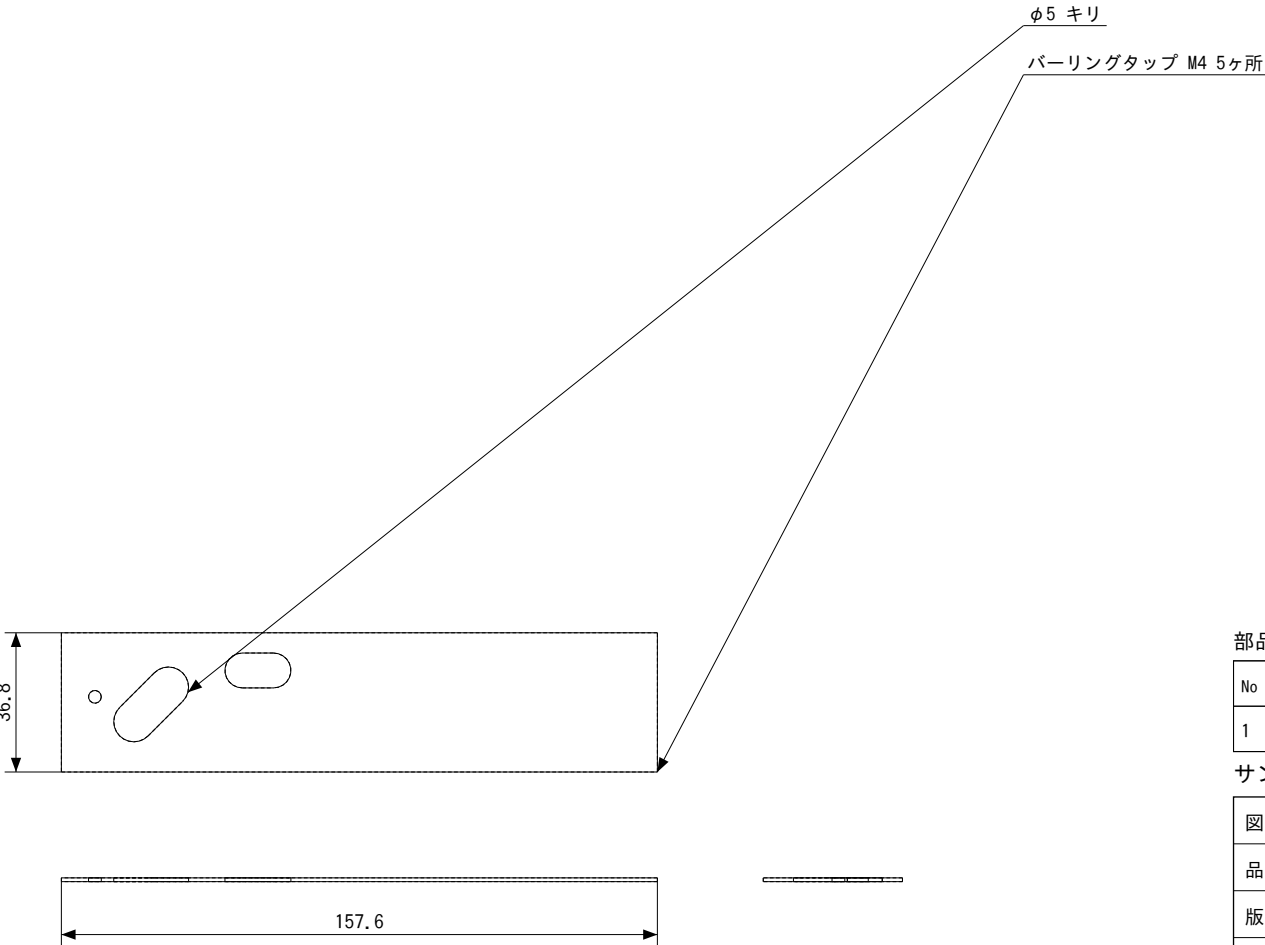
展開図（参考）
