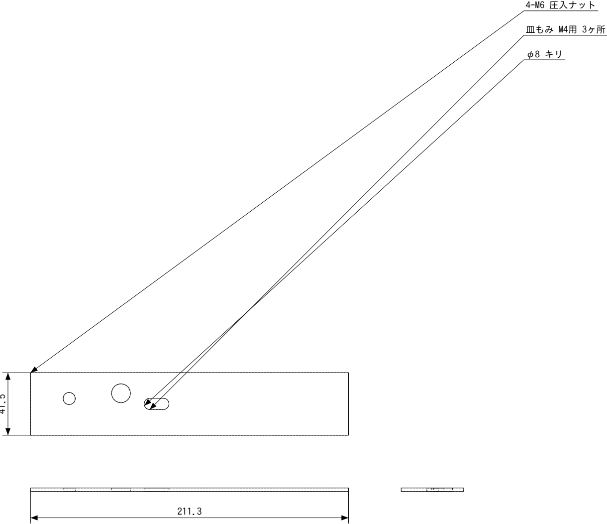
展開図（参考）
